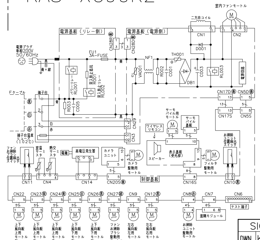
配線図 RAS-XC90K2
