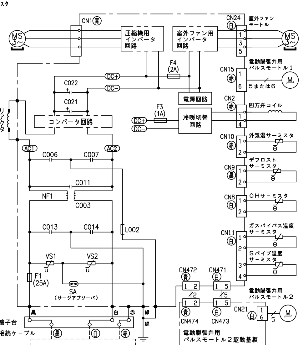
配線図 RAC-XC90K2
