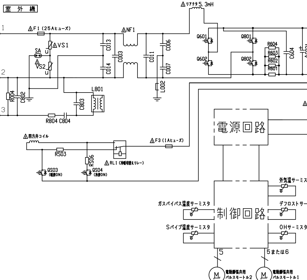
配線図 RAS-XC90K2
