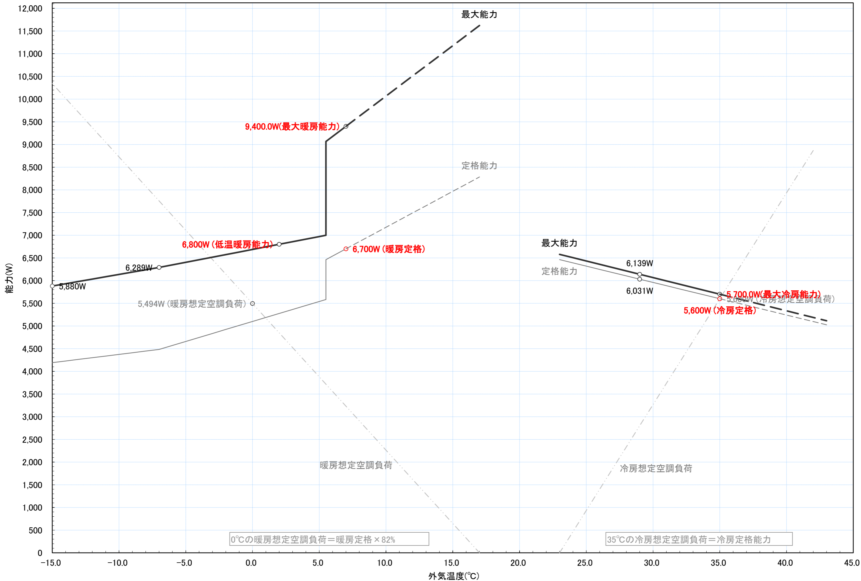
RAP-56M2 冷暖房能力特性図 [室温 冷房:27°C一定, 暖房:20°C一定]
