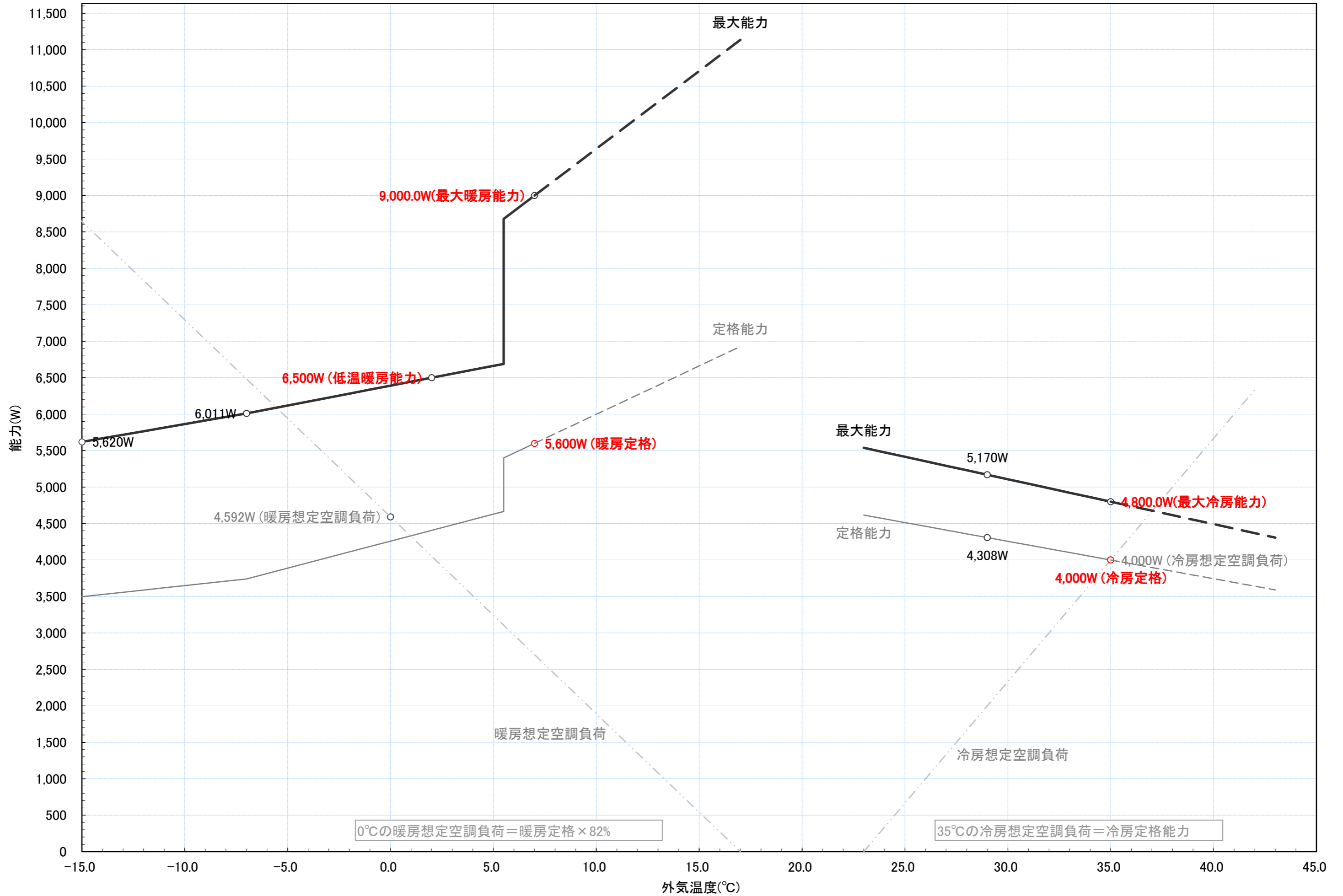
RAP-40M2 冷暖房能力特性図 [室温 冷房:27°C一定, 暖房:20°C一定]
