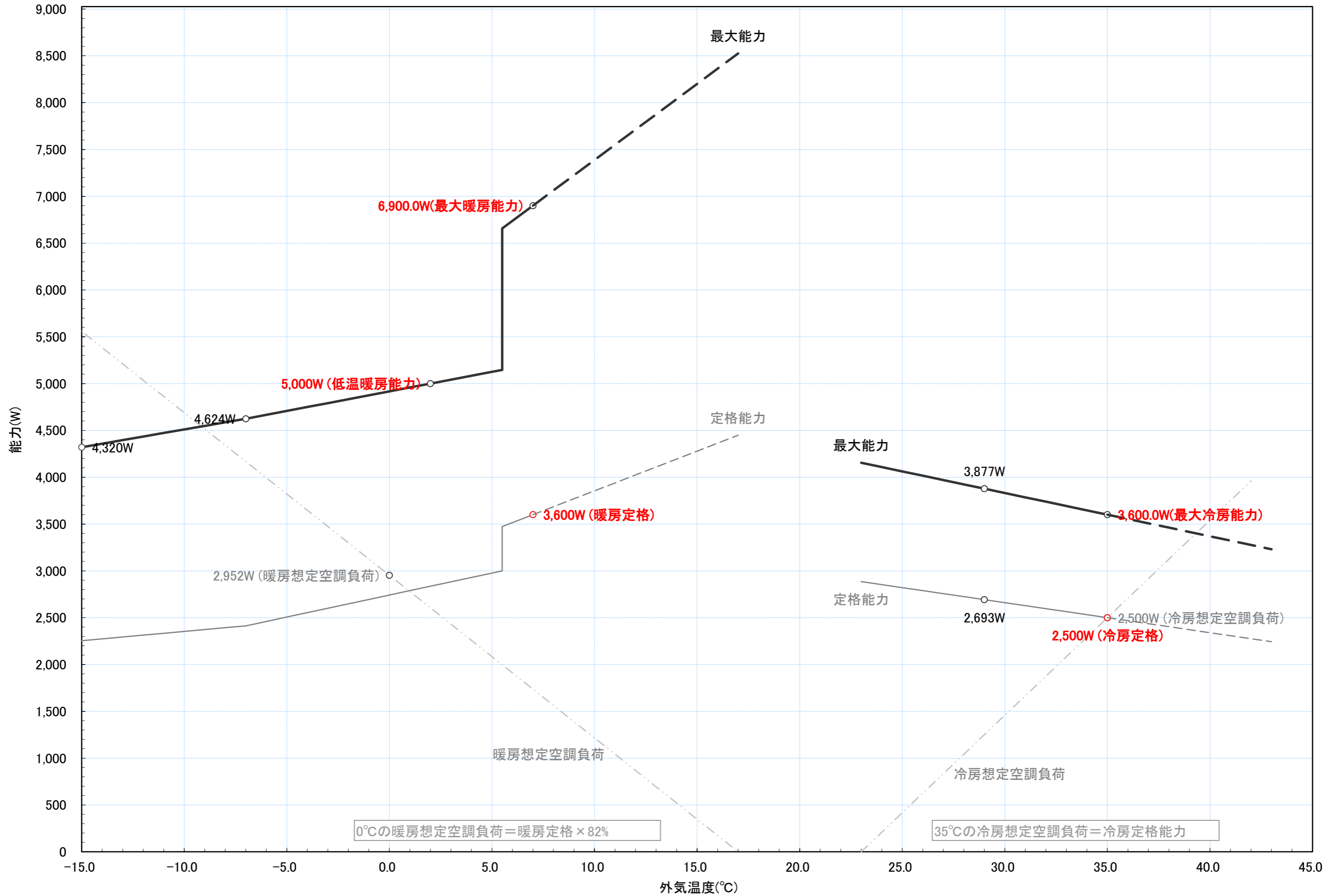
RAP-25M2 冷暖房能力特性図 [室温 冷房:27°C一定, 暖房:20°C一定]
