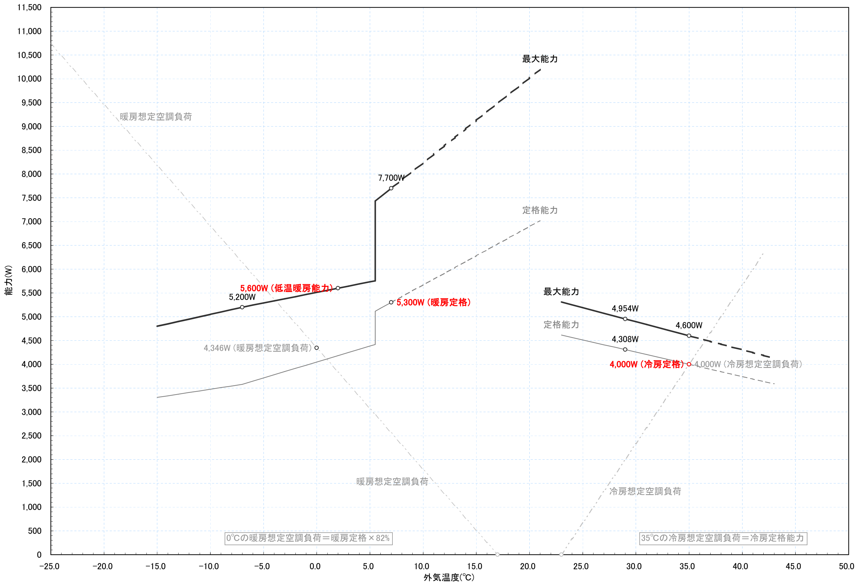
RAJ-40D2 冷暖房能力特性図 [室温 冷房:27°C一定, 暖房:20°C一定]
