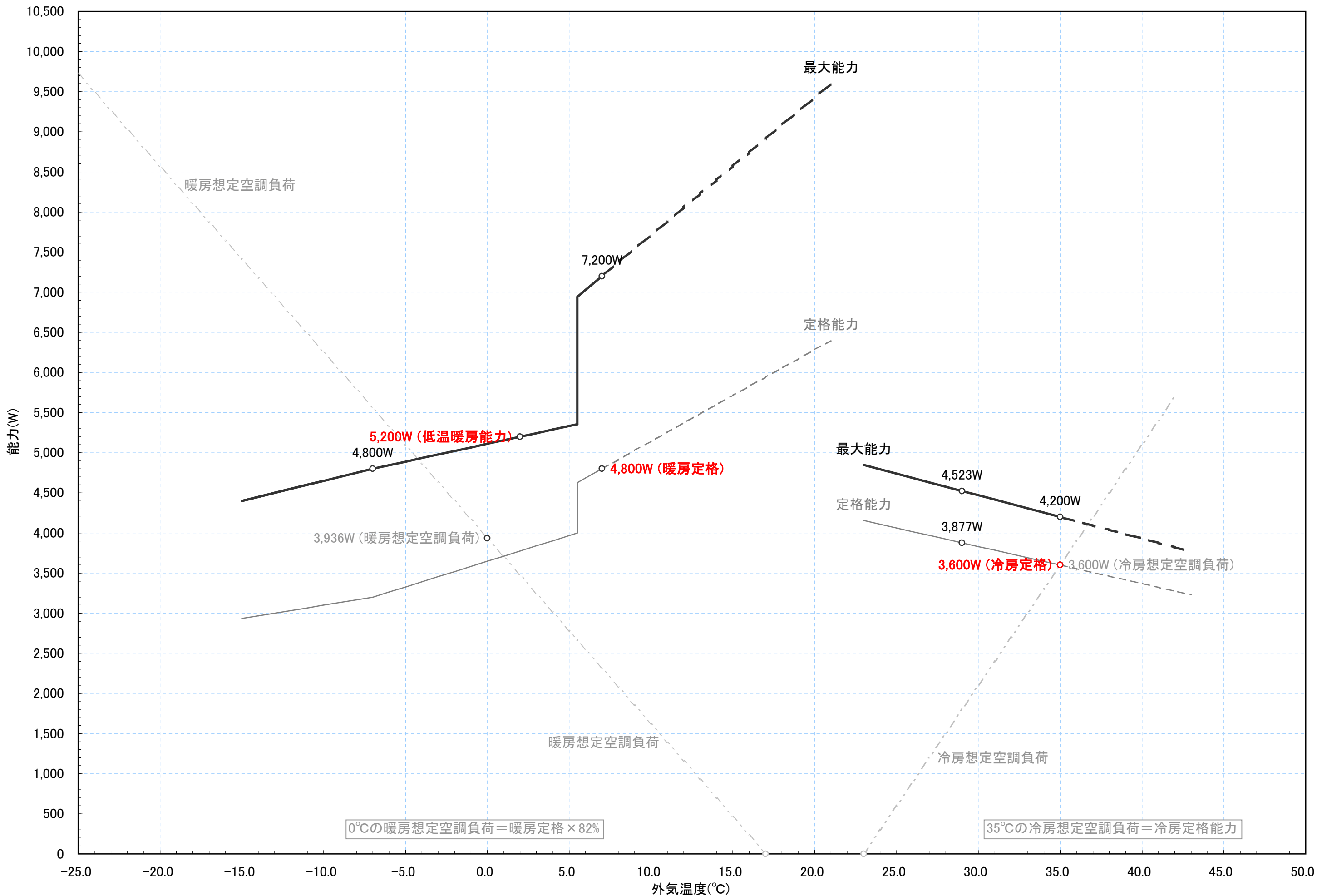
RAJ-36D2 冷暖房能力特性図 [室温 冷房:27°C一定, 暖房:20°C一定]
