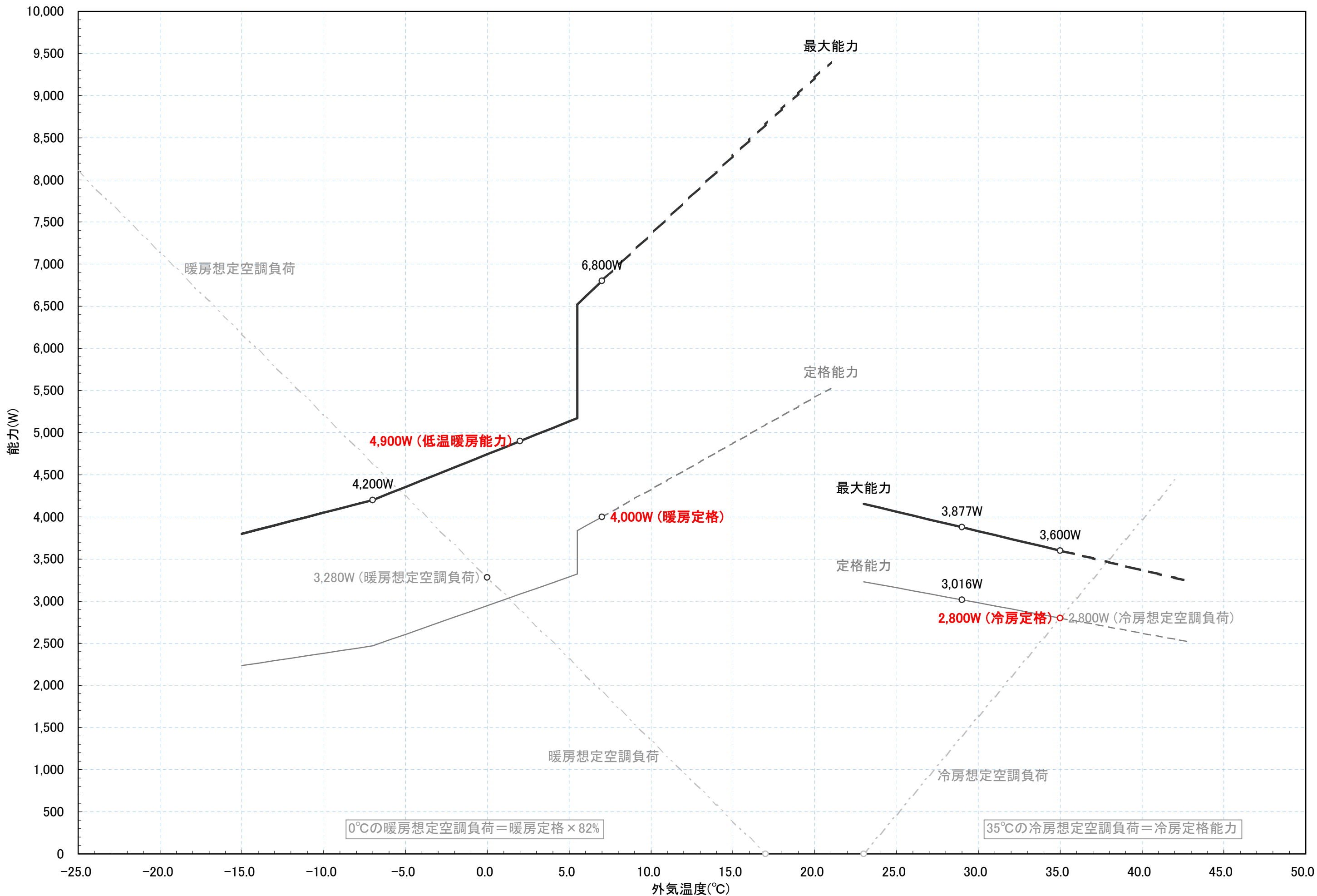
RAJ-28D2 冷暖房能力特性図 [室温 冷房:27°C一定, 暖房:20°C一定]
