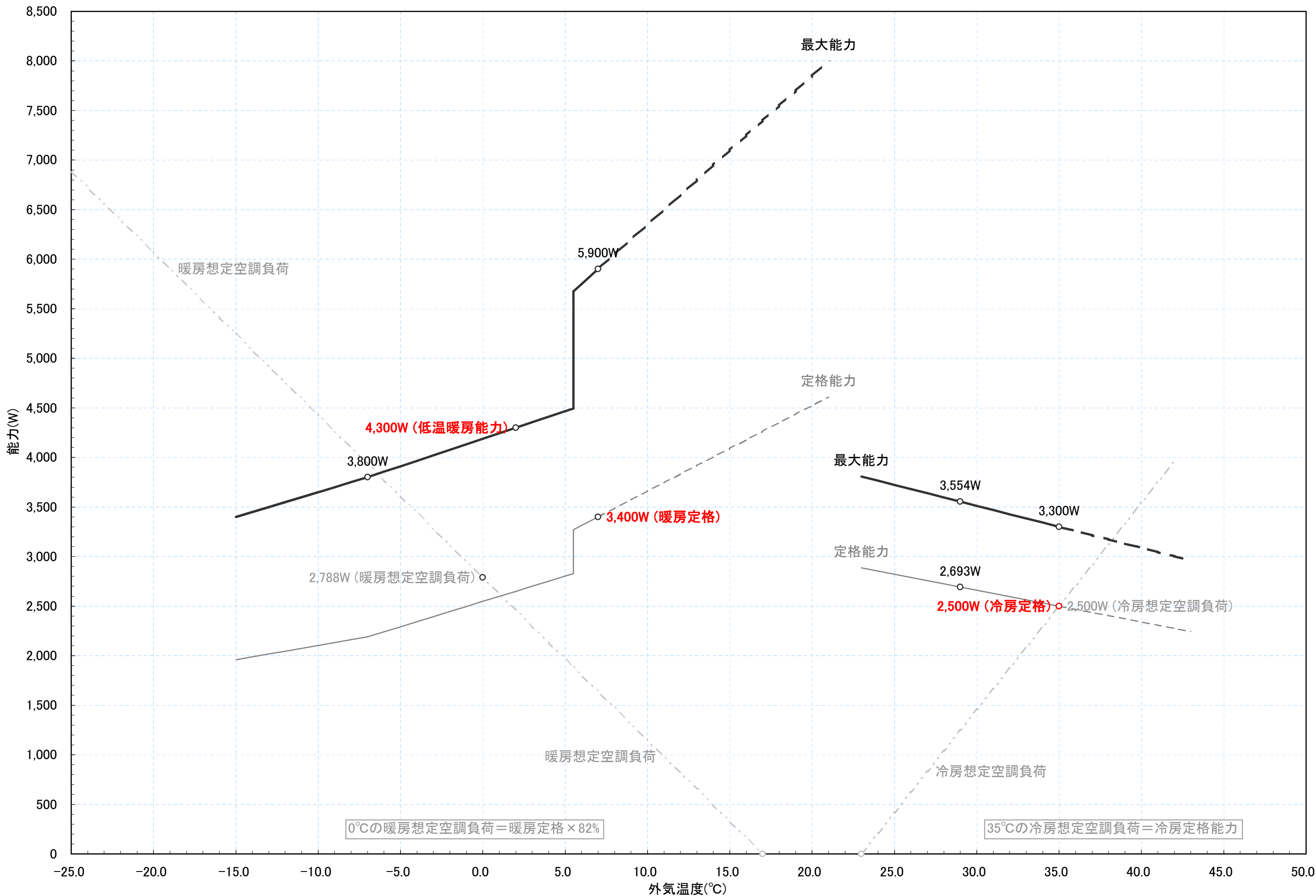
RAJ-25D2 冷暖房能力特性図 [室温 冷房:27°C一定, 暖房:20°C一定]
