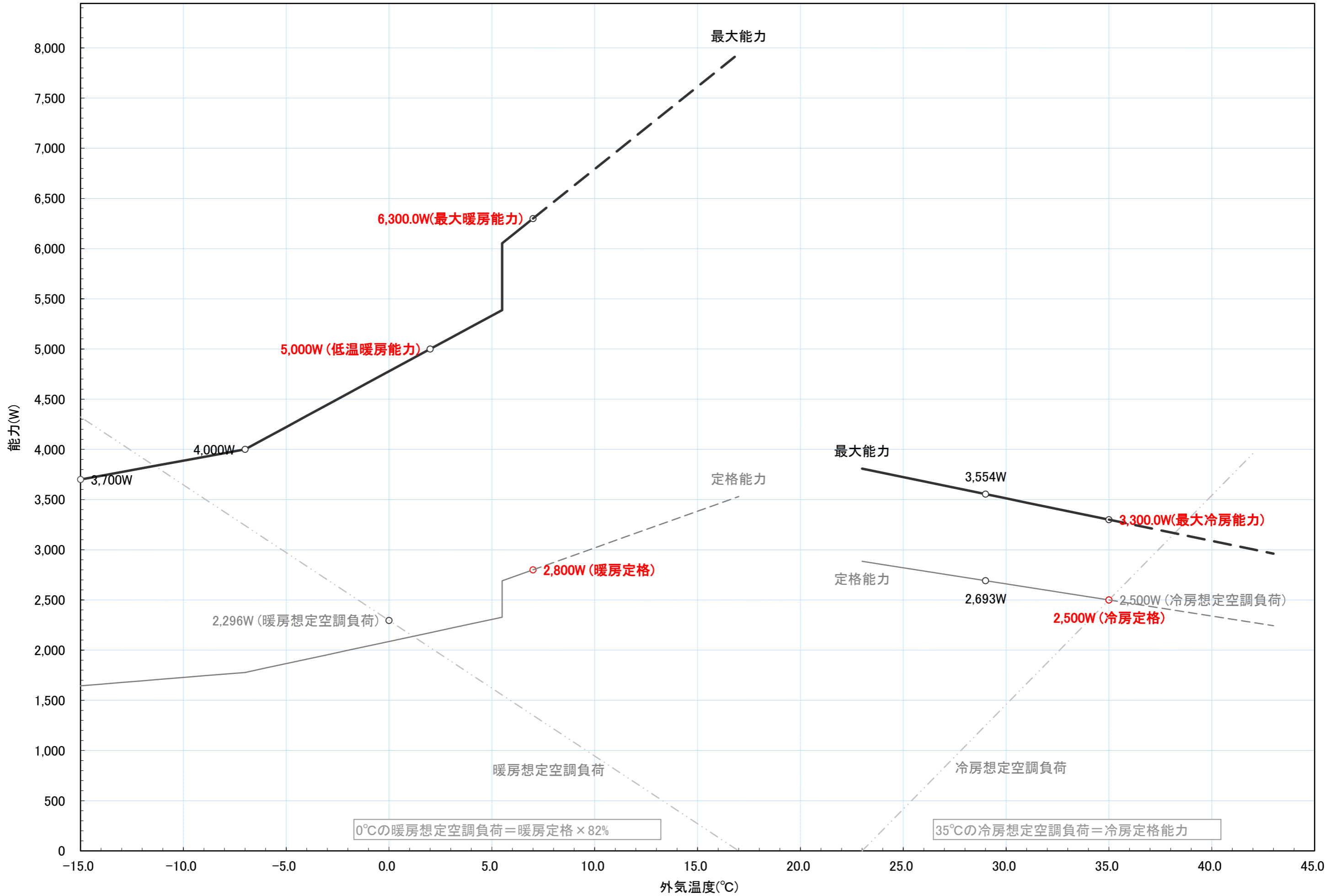
RAS-RK25R 冷暖房能力特性図 [室温 冷房:27°C一定, 暖房:20°C一定]
