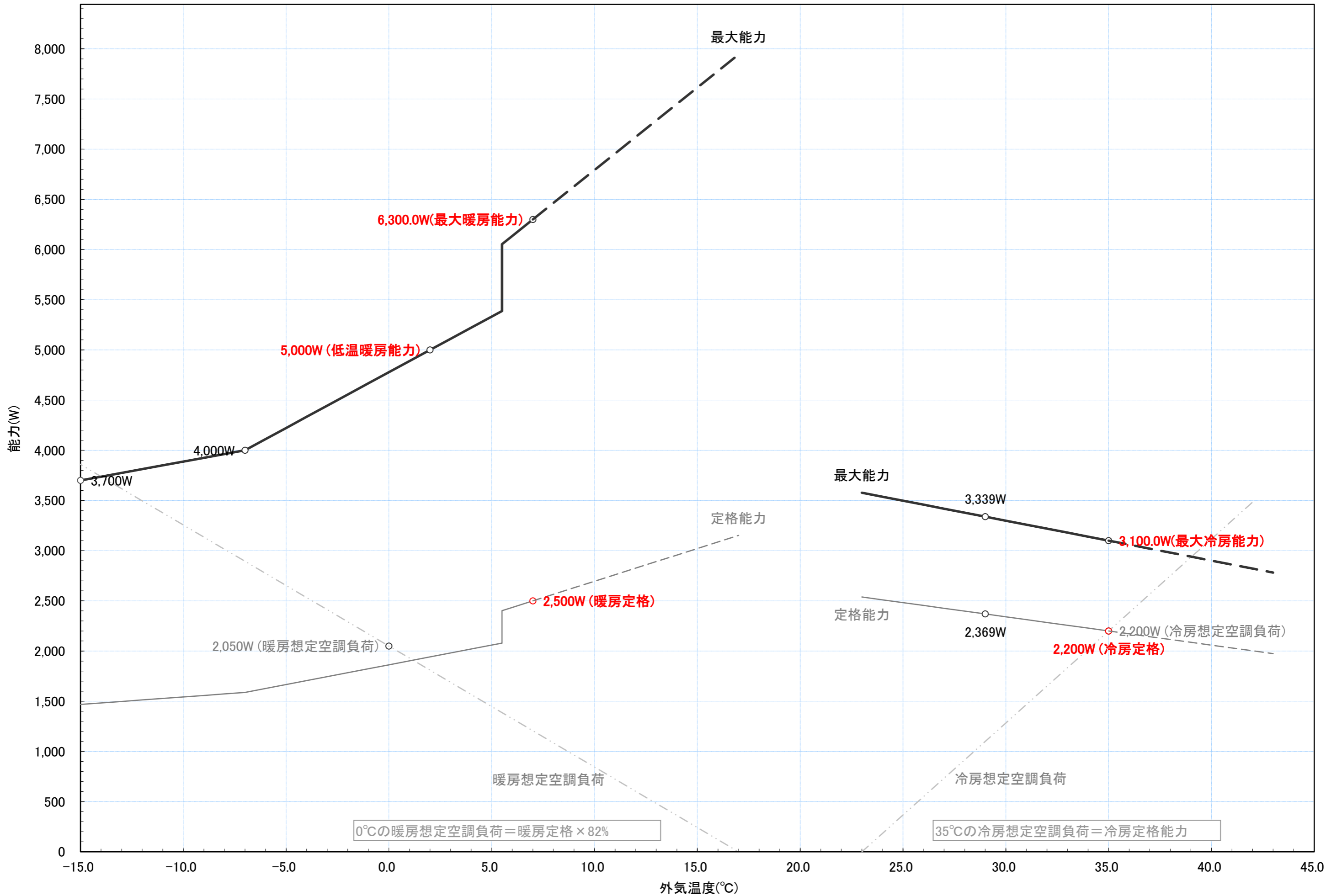
RAS-RK22R 冷暖房能力特性図 [室温 冷房:27°C一定, 暖房:20°C一定]
