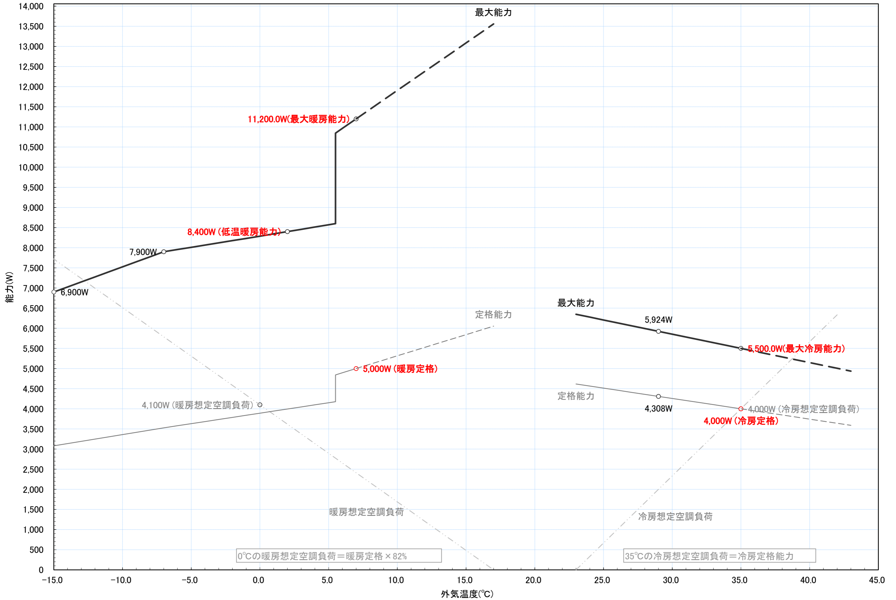
RAS-EK40R2 冷暖房能力特性図 [室温 冷房:27°C一定, 暖房:20°C一定]
