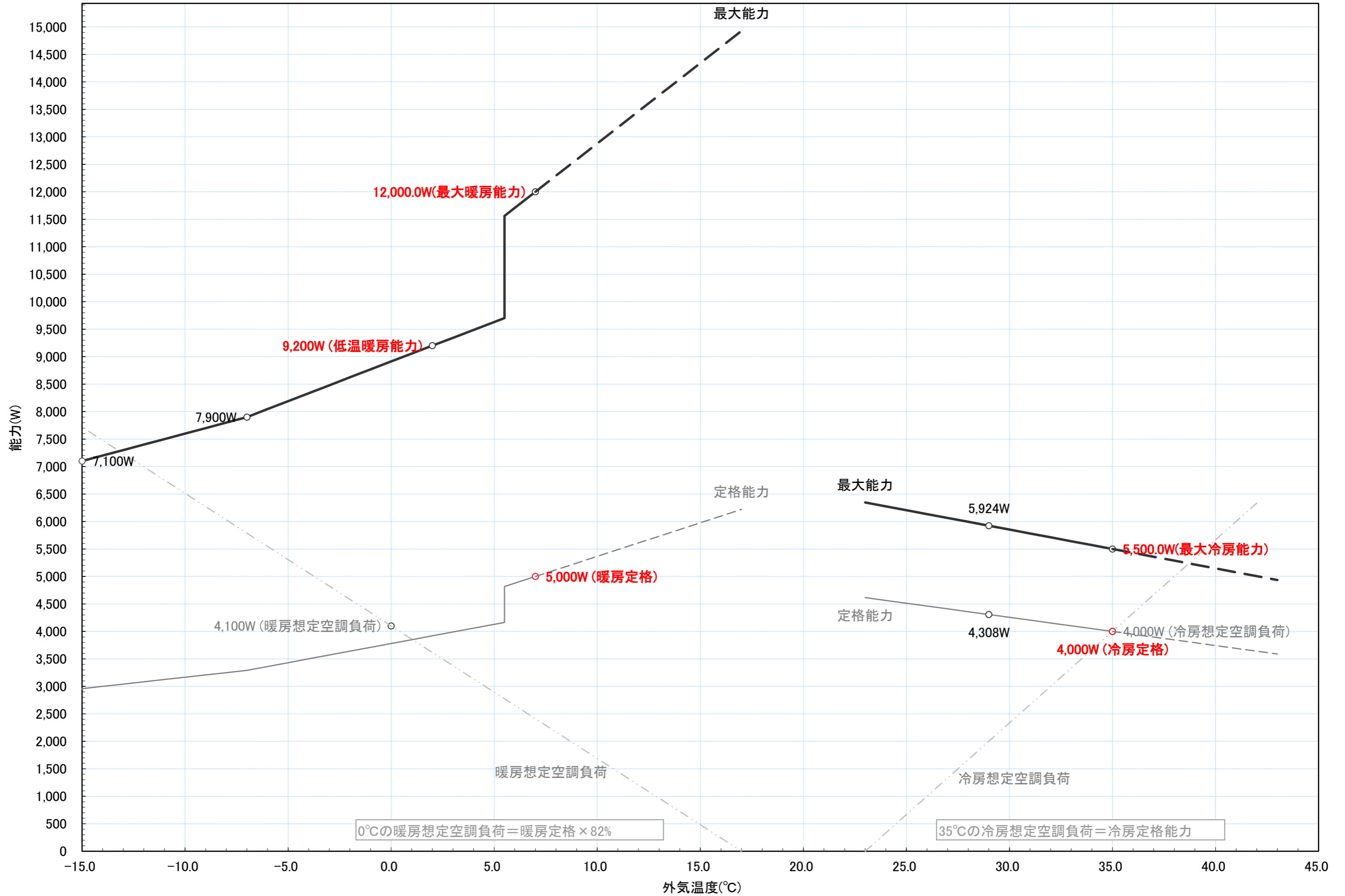
RAS-XK40N2 冷暖房能力特性図 [室温 冷房:27°C一定, 暖房:20°C一定]
