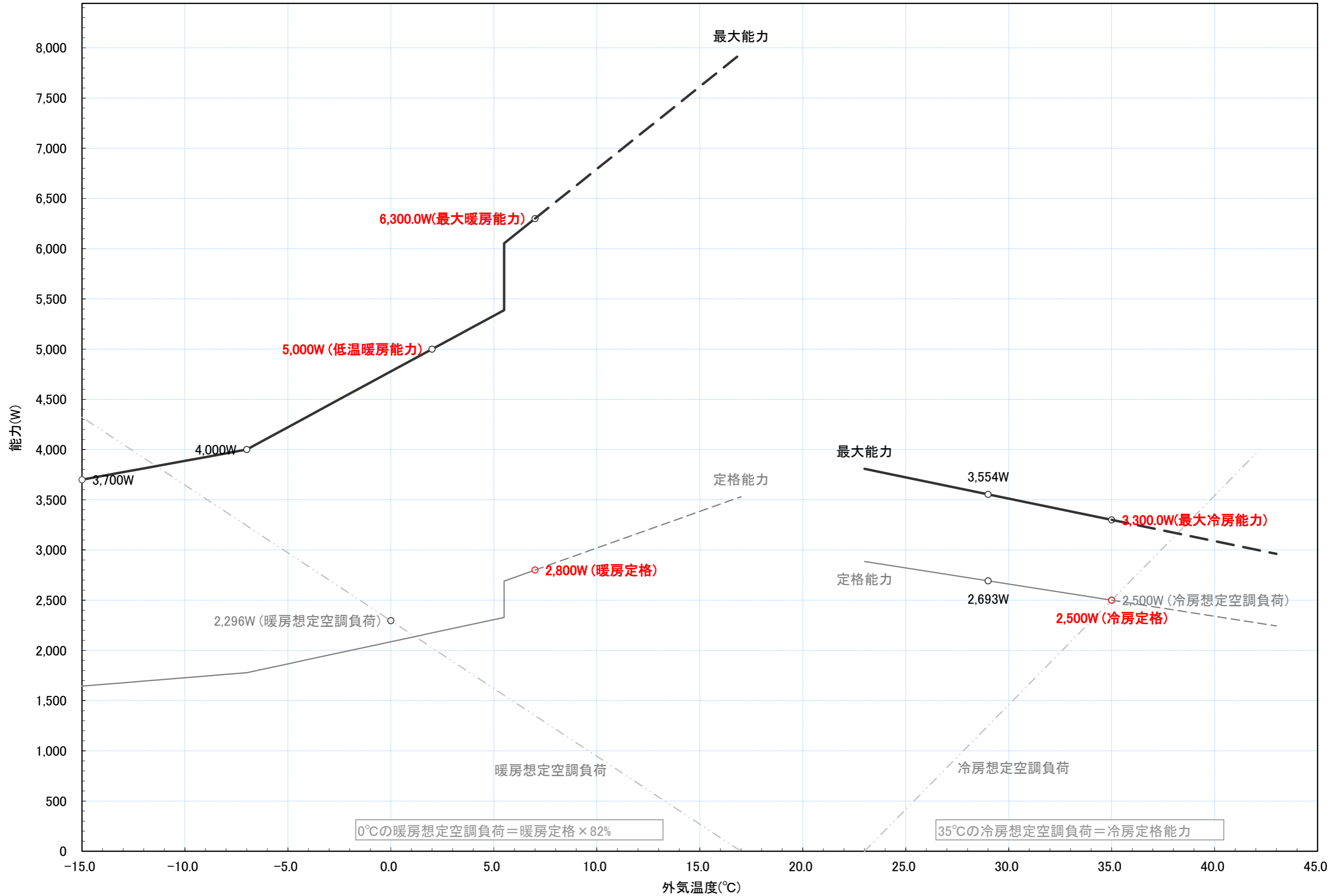
RAS-RK25N 冷暖房能力特性図 [室温 冷房:27°C一定, 暖房:20°C一定]
