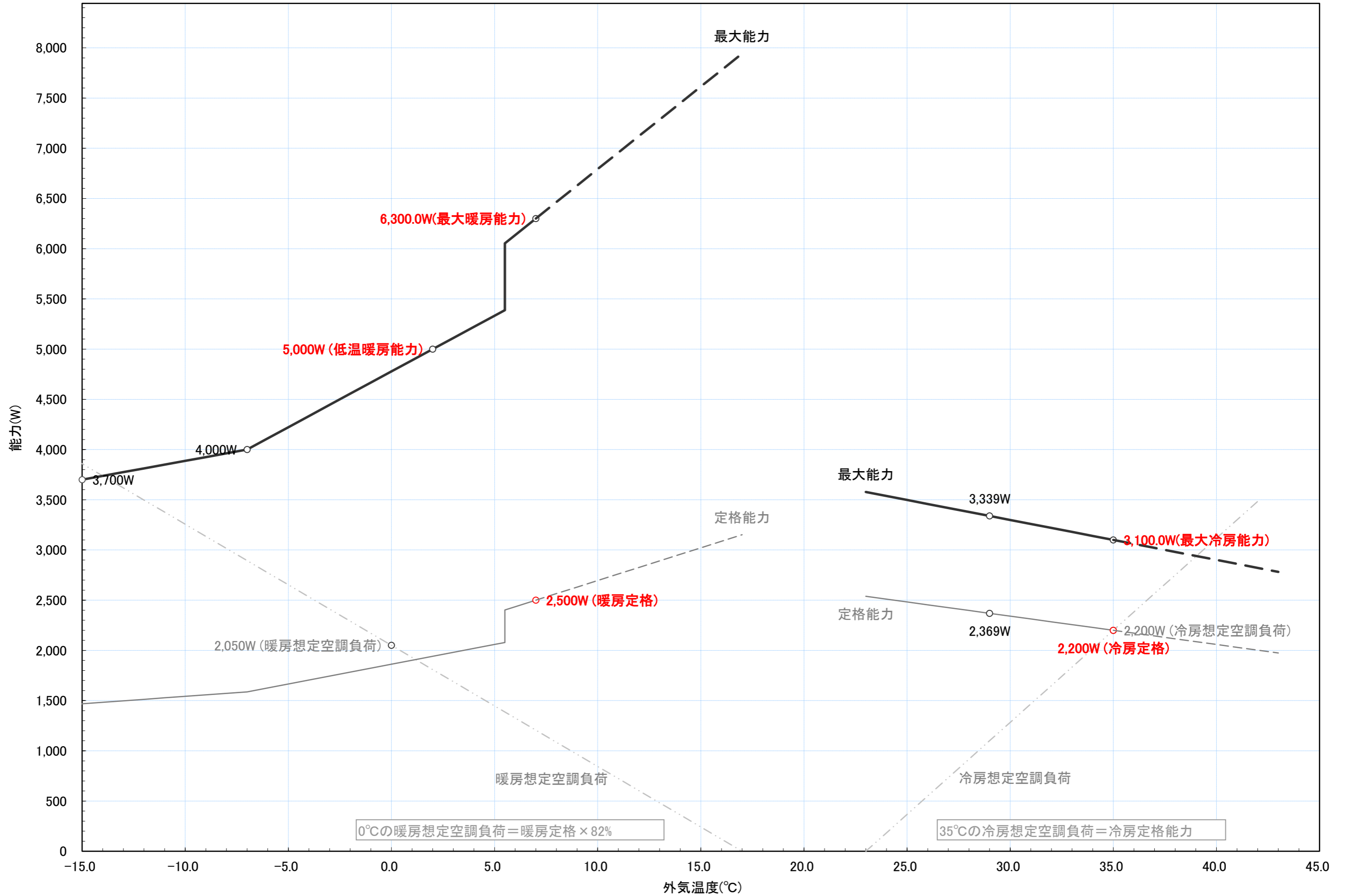
RAS-RK22N 冷暖房能力特性図 [室温 冷房:27°C一定, 暖房:20°C一定]
