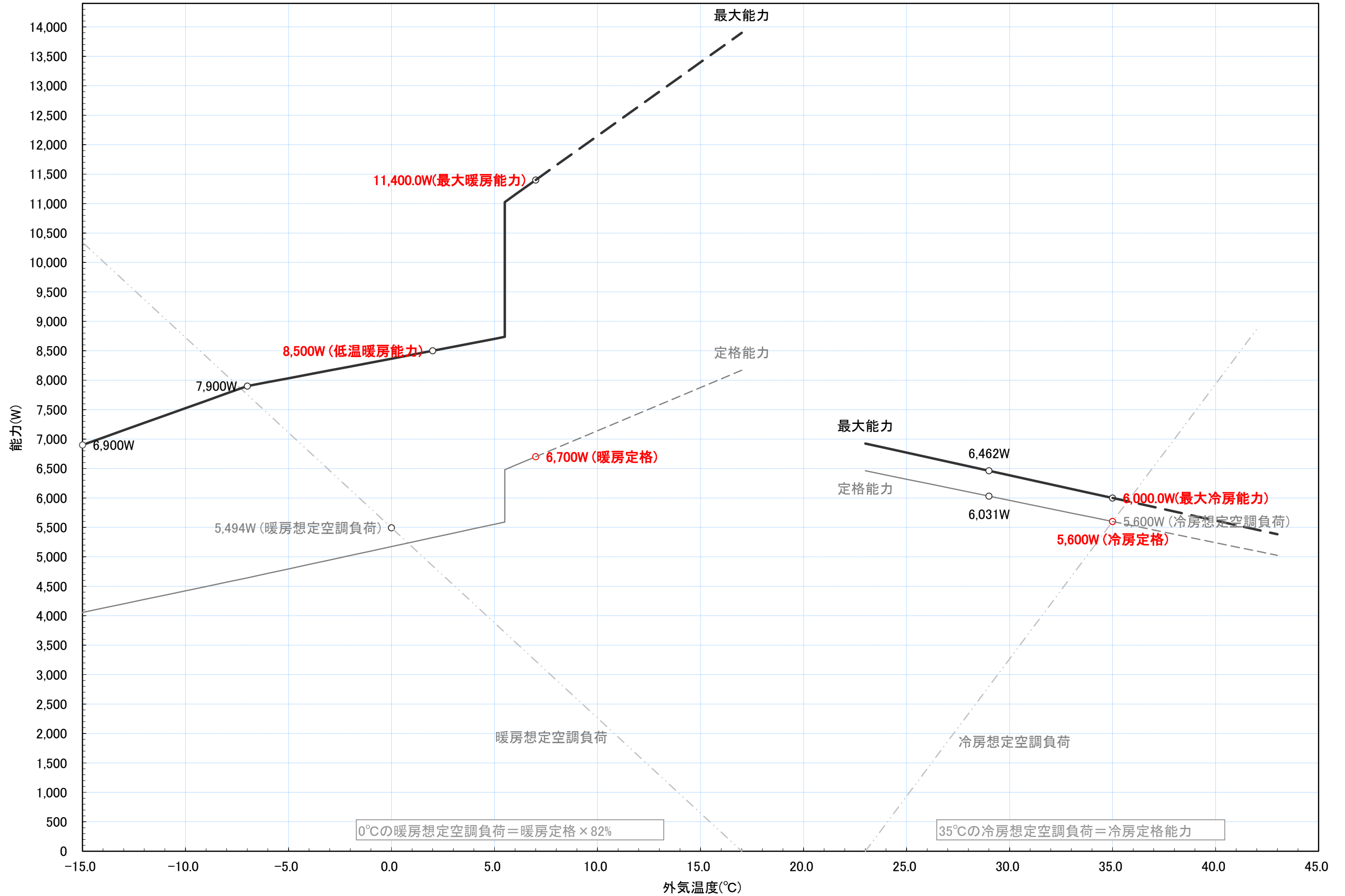
RAS-EK56N2 冷暖房能力特性図 [室温 冷房:27°C一定, 暖房:20°C一定]
