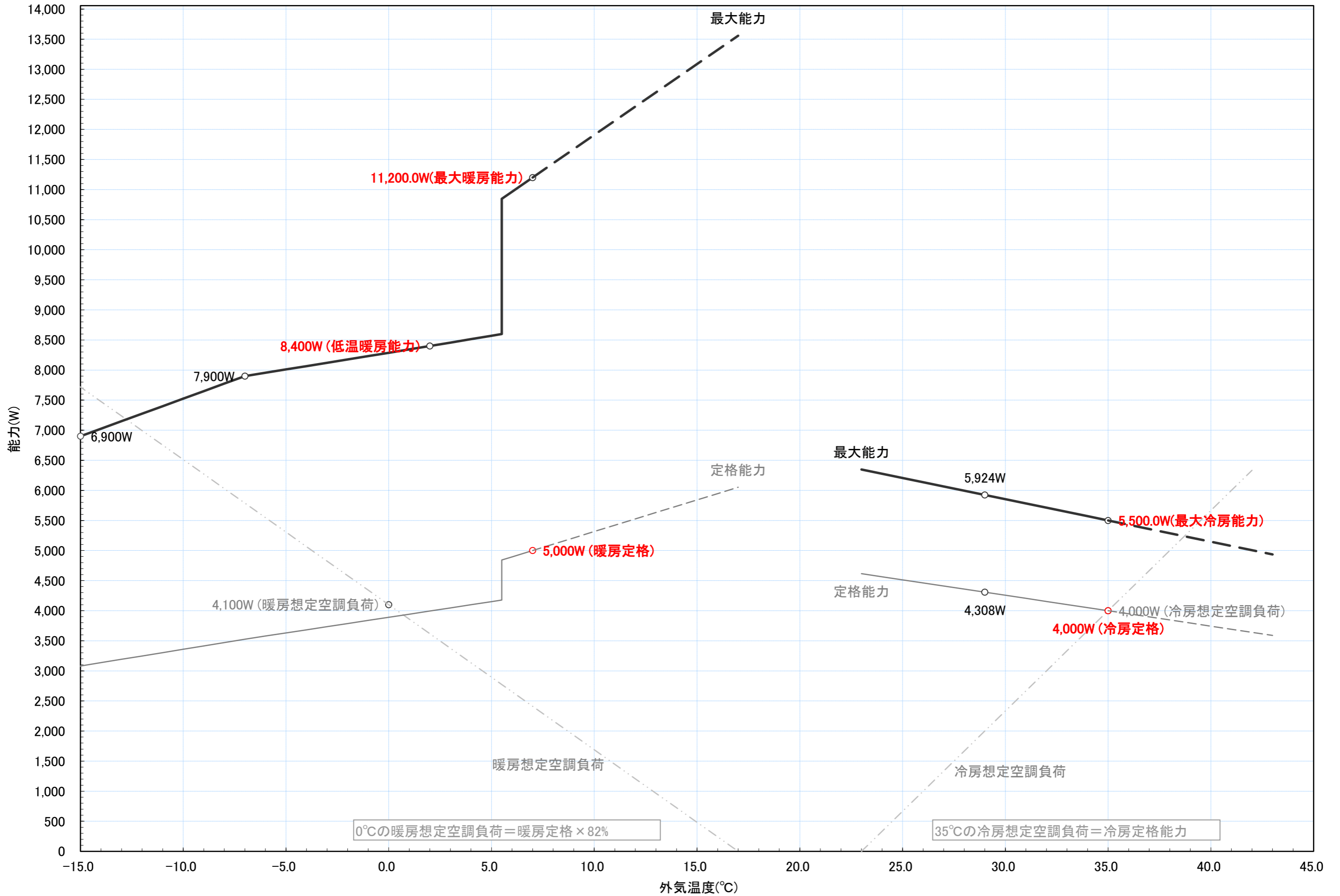
RAS-EK40N2 冷暖房能力特性図 [室温 冷房:27°C一定, 暖房:20°C一定]
