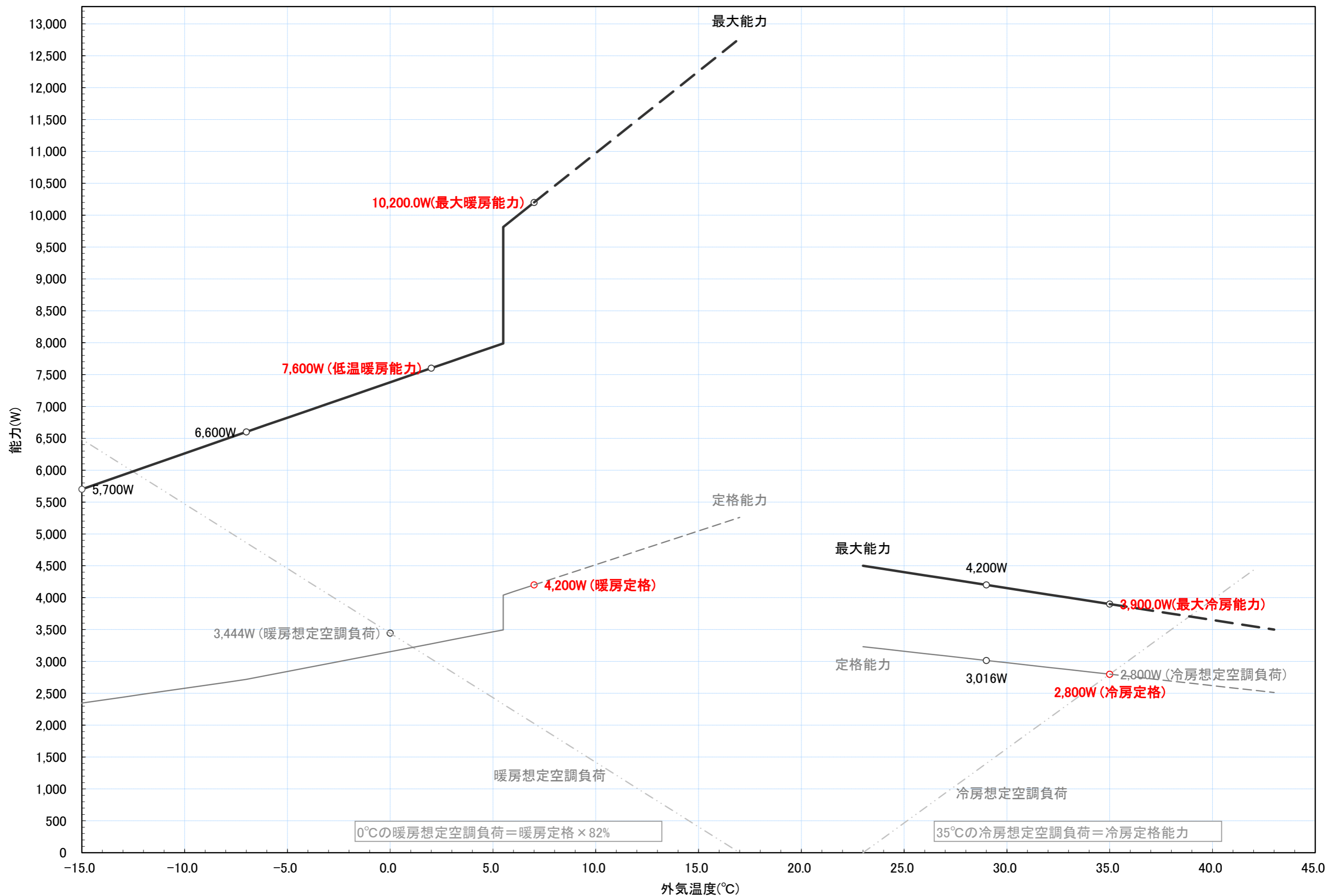
RAS-EK28N2 冷暖房能力特性図 [室温 冷房:27°C一定, 暖房:20°C一定]
