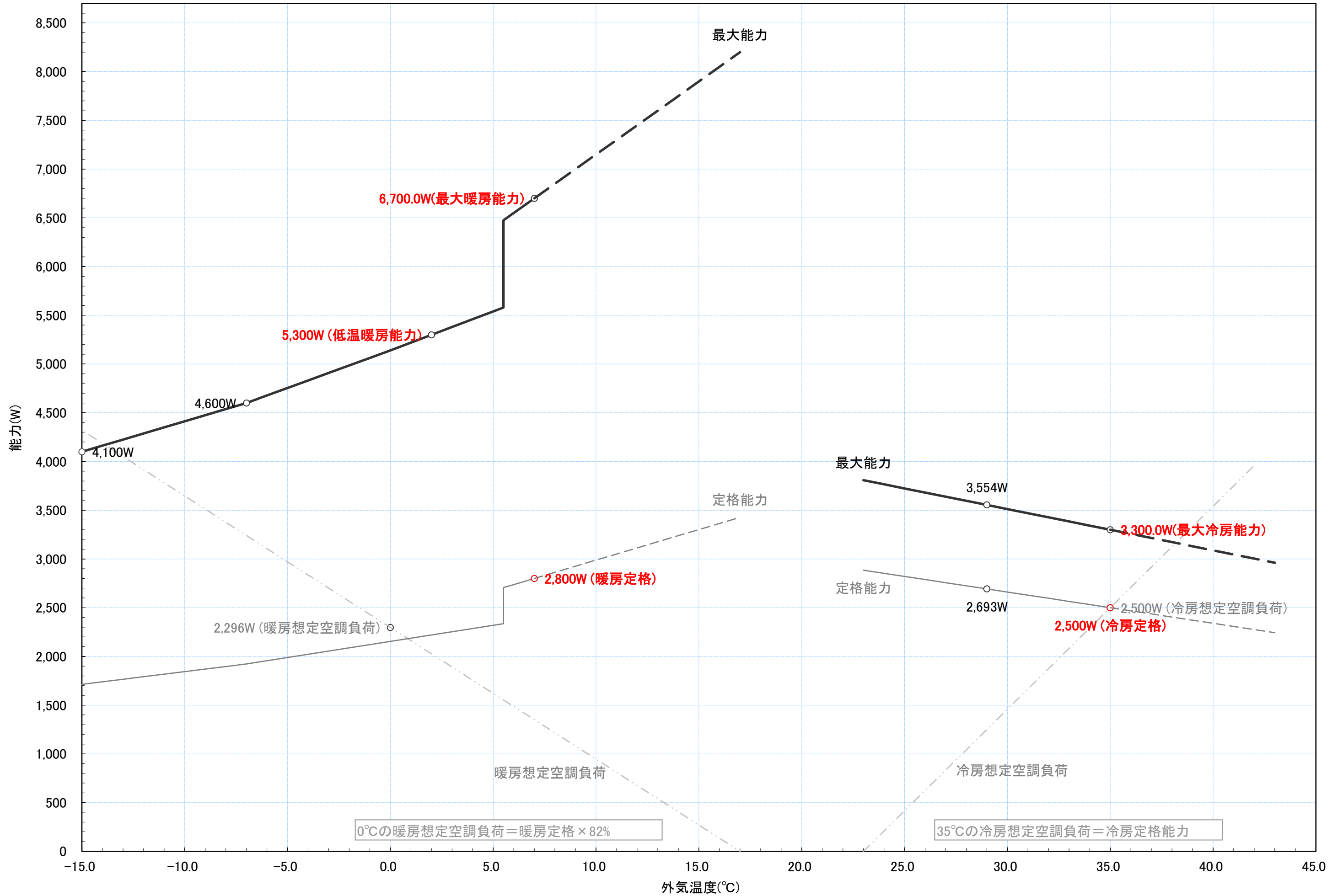
RAS-HK25L 冷暖房能力特性図 [室温 冷房:27°C一定, 暖房:20°C一定]
