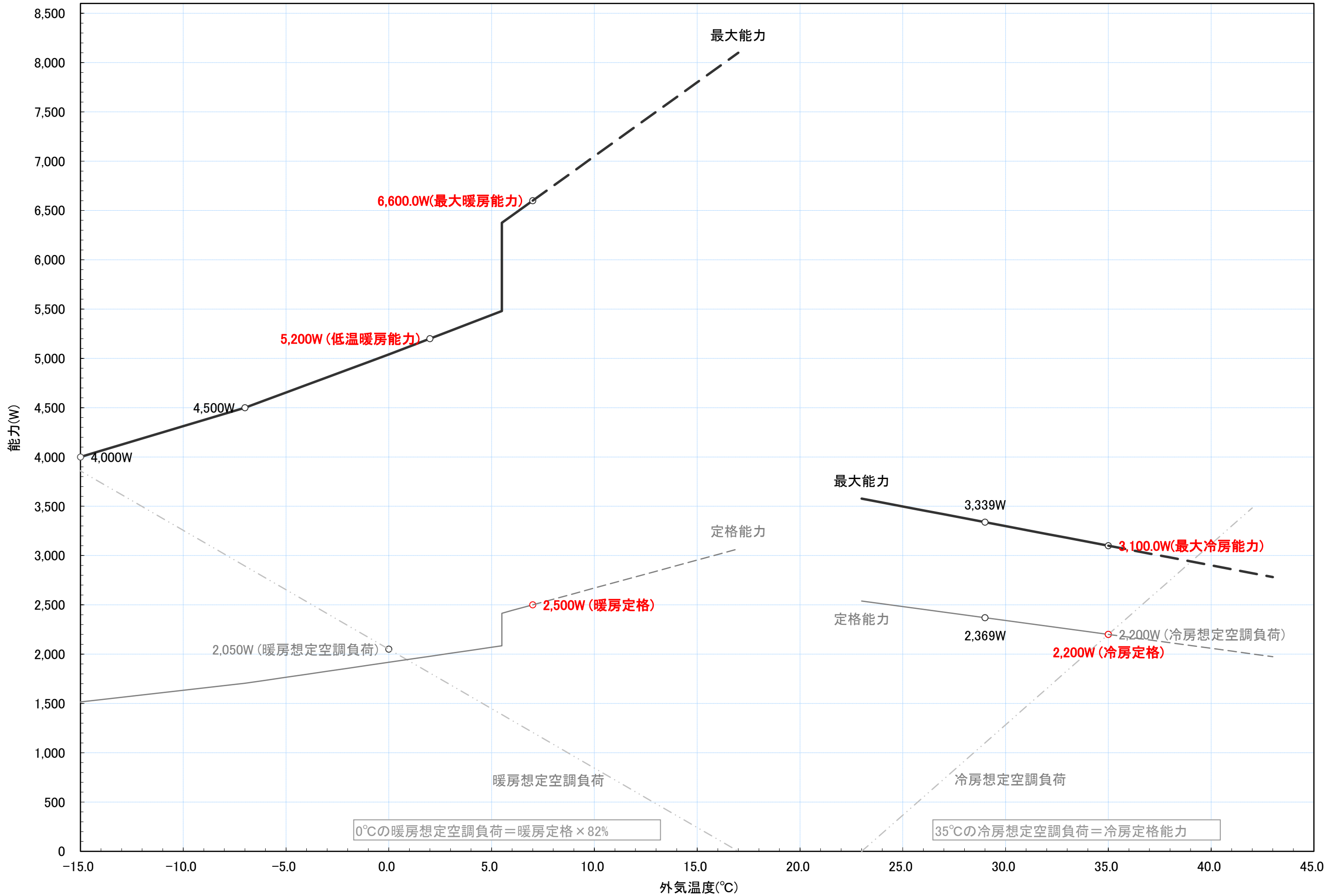
RAS-HK22L 冷暖房能力特性図 [室温 冷房:27°C一定, 暖房:20°C一定]
