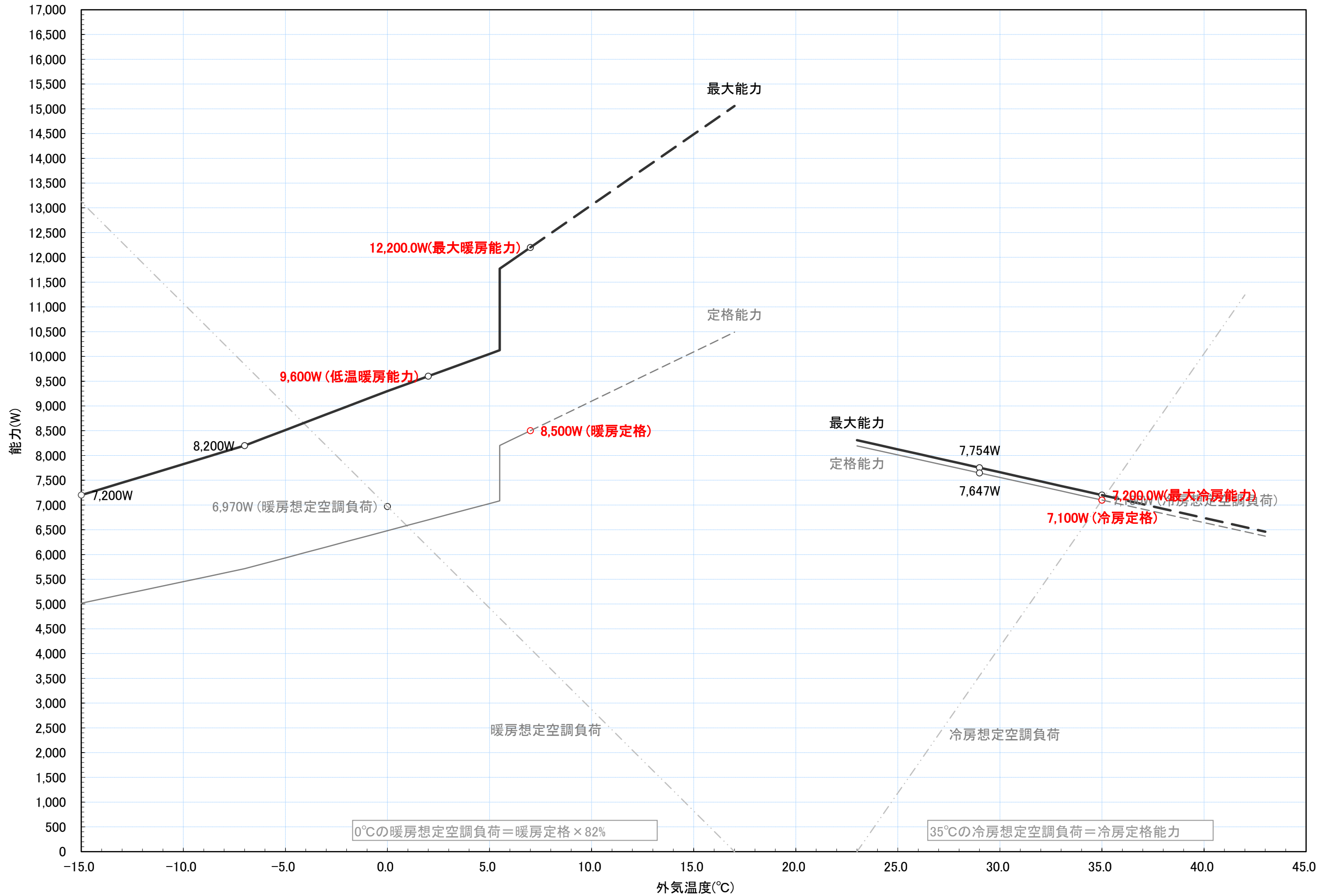
RAS-XK71K2 冷暖房能力特性図 [室温 冷房:27°C一定, 暖房:20°C一定]
