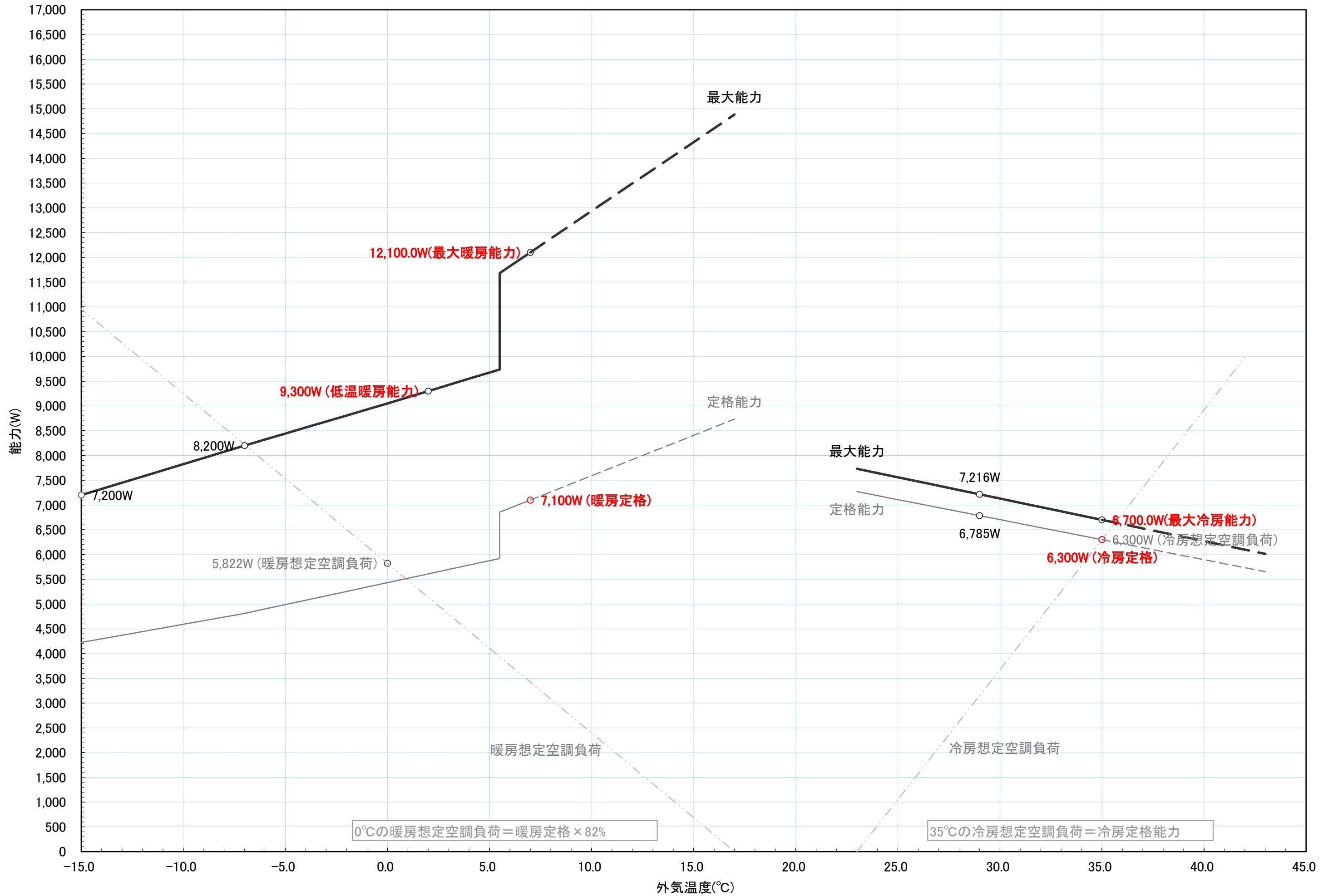
RAS-XK63K2 冷暖房能力特性図 [室温 冷房:27°C一定, 暖房:20°C一定]
