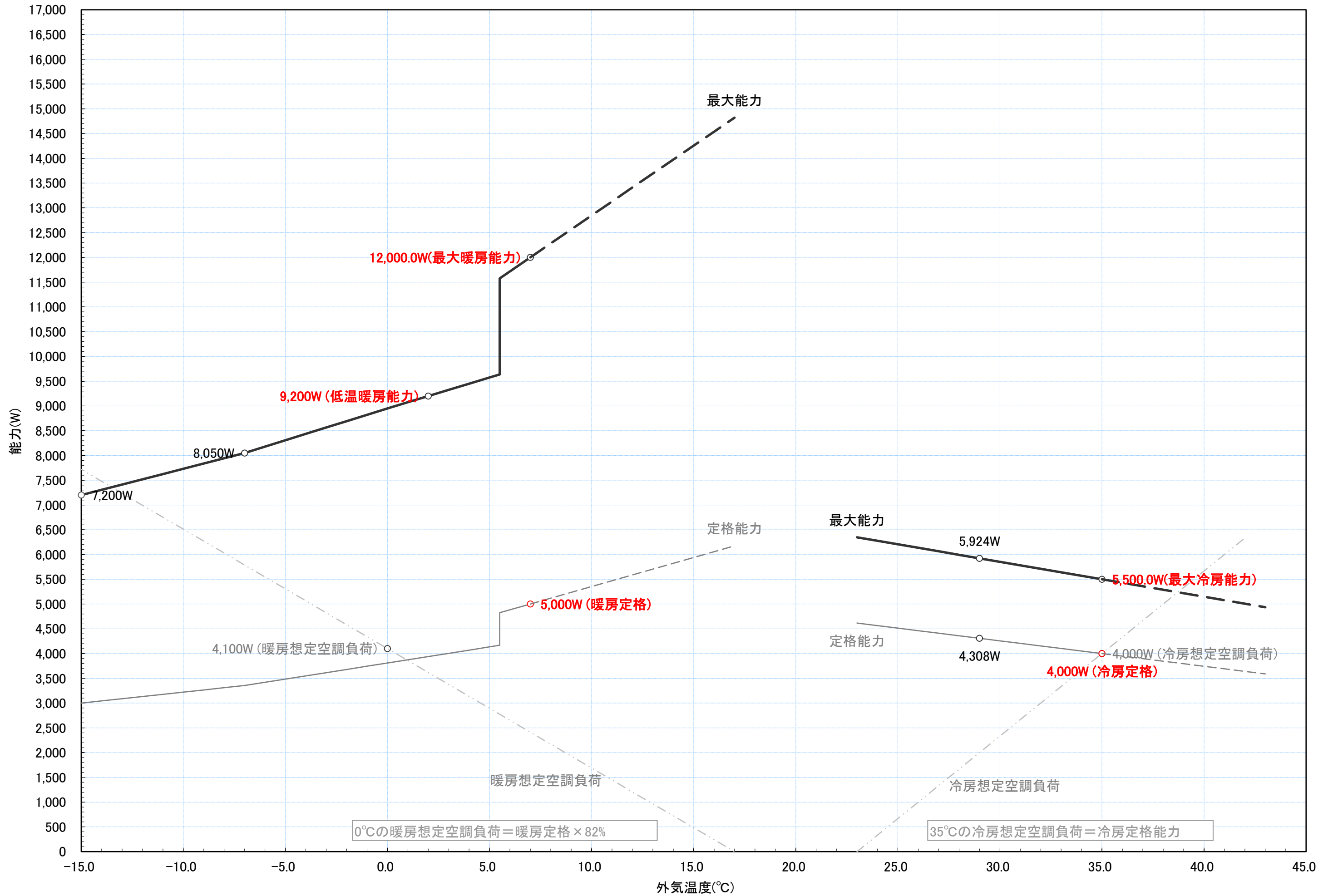
RAS-XK40K2 冷暖房能力特性図 [室温 冷房:27°C一定, 暖房:20°C一定]
