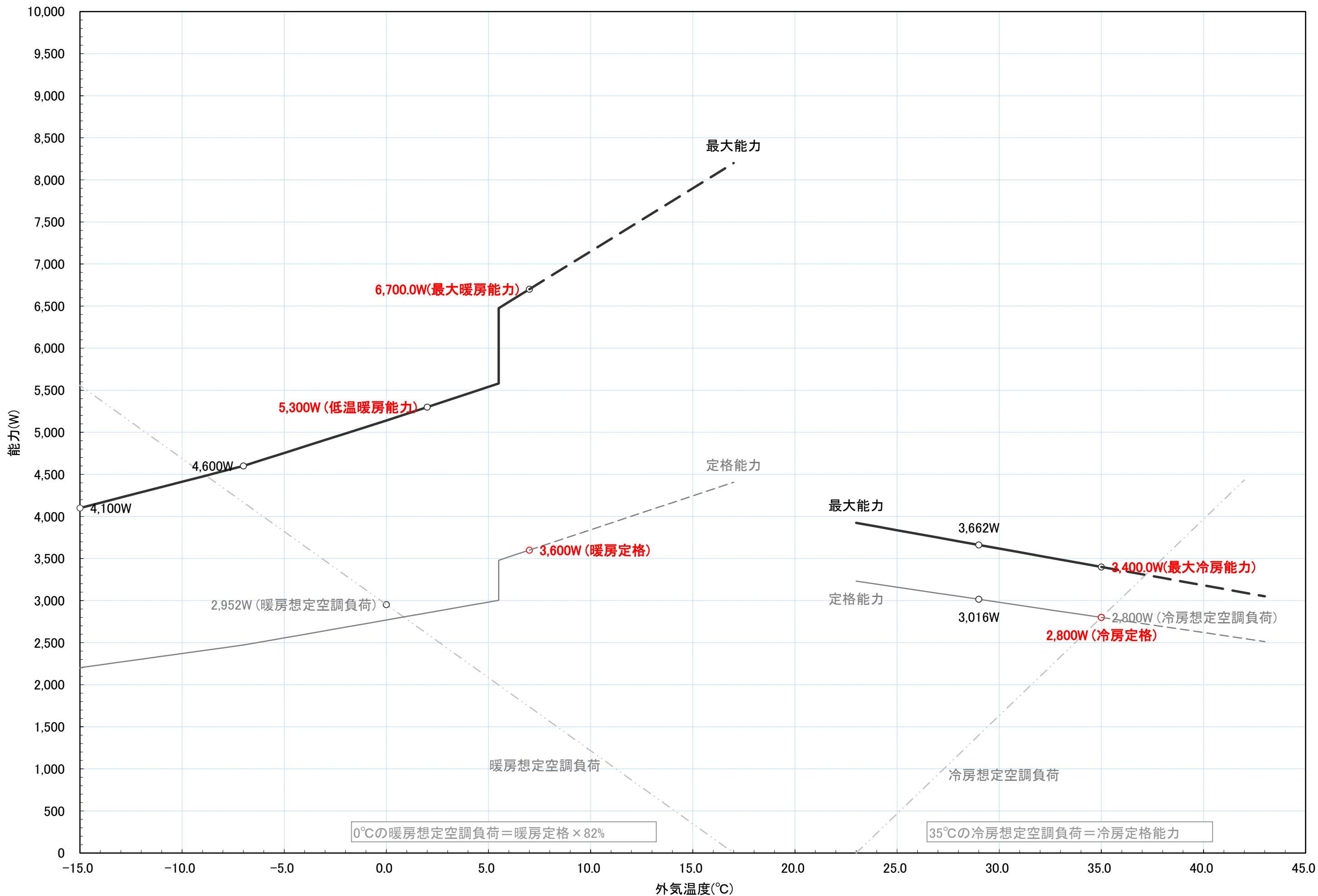
RAS-HK28K 冷暖房能力特性図 [室温 冷房:27°C一定, 暖房:20°C一定]
