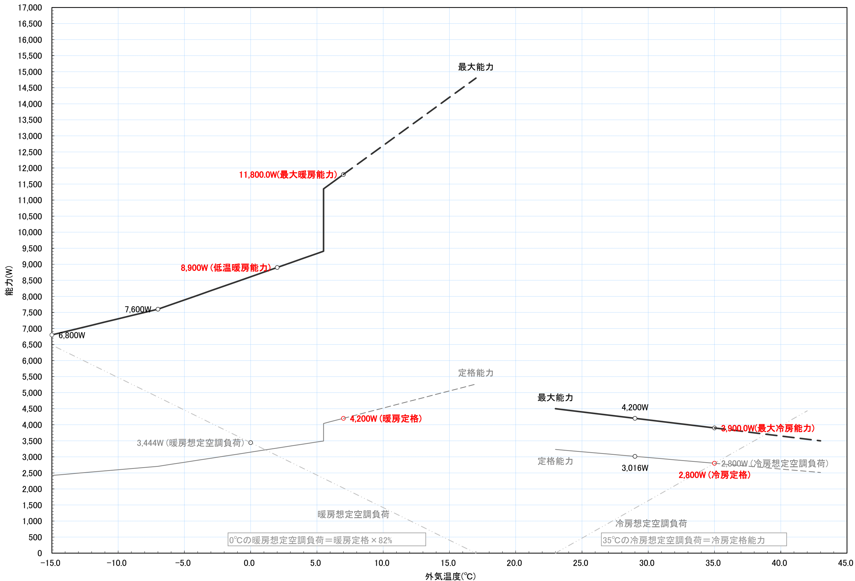
RAS-XK28J2 冷暖房能力特性図 [室温 冷房:27°C一定, 暖房:20°C一定]
