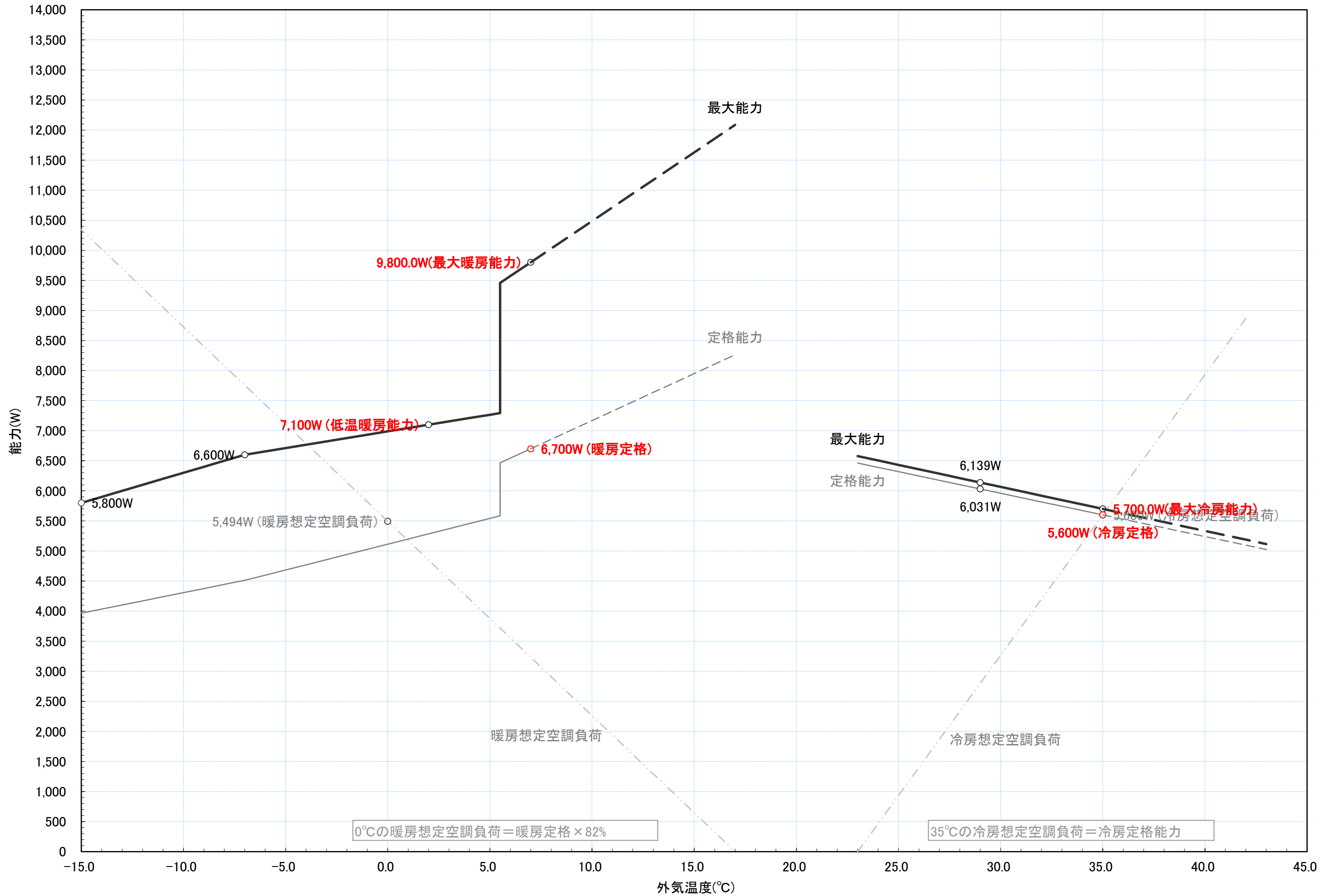
RAP-K56J2 冷暖房能力特性図 [室温 冷房:27°C一定, 暖房:20°C一定]
