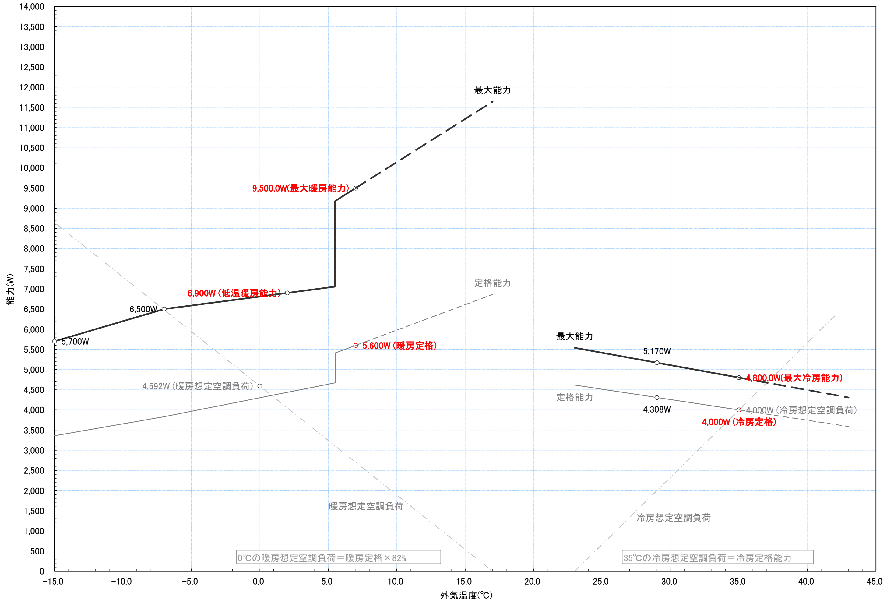
RAP-K40J2 冷暖房能力特性図 [室温 冷房:27°C一定, 暖房:20°C一定]
