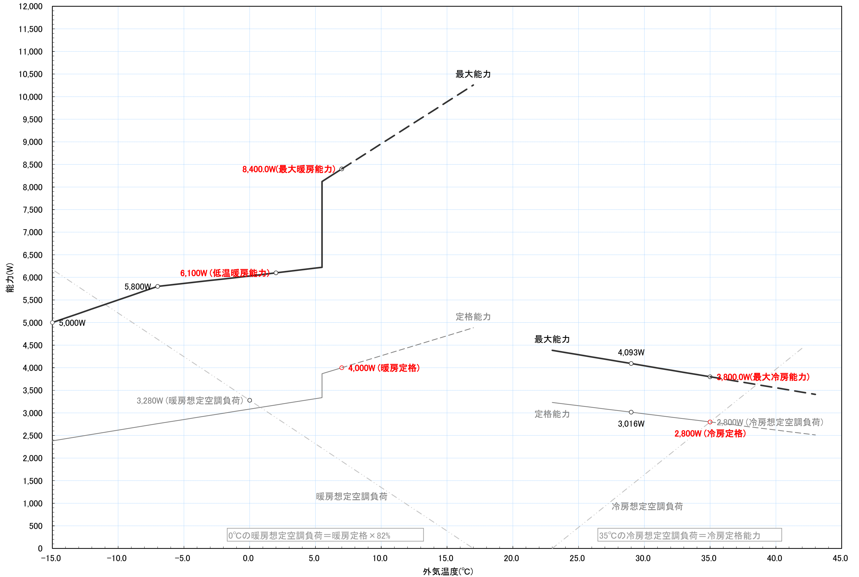
RAP-K28J2 冷暖房能力特性図 [室温 冷房:27°C一定, 暖房:20°C一定]
