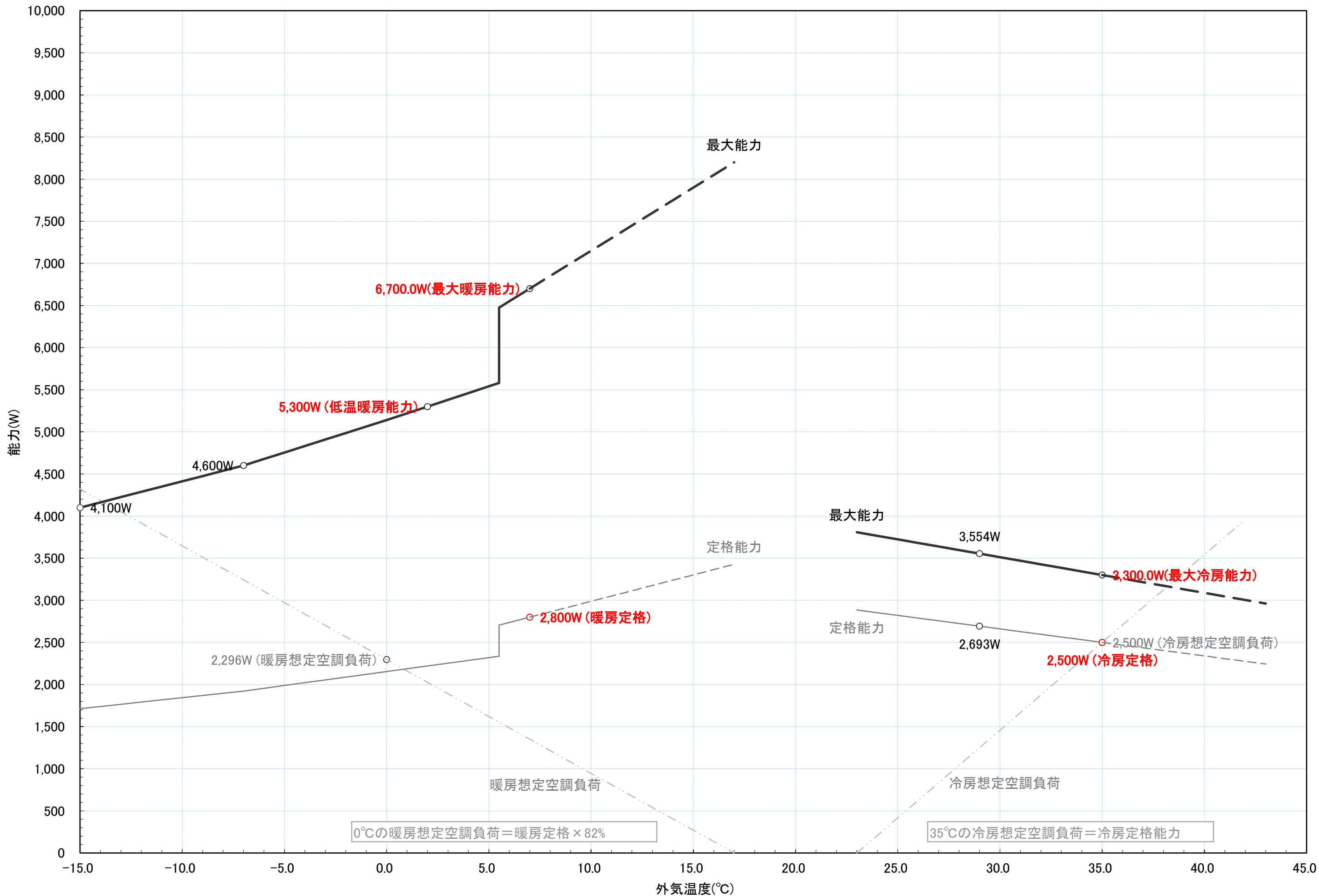
RAS-HK25J 冷暖房能力特性図 [室温 冷房:27°C一定, 暖房:20°C一定]
