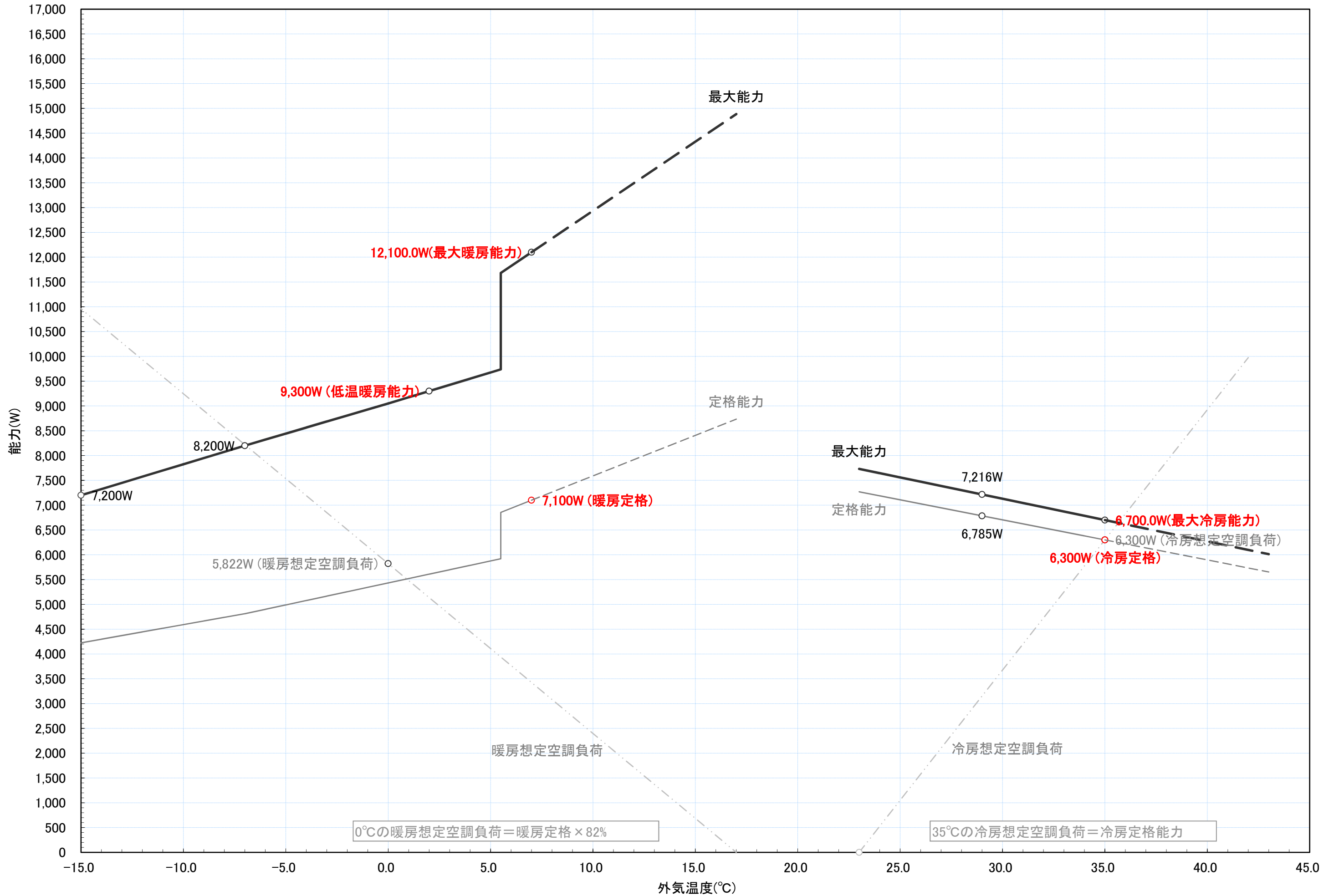
RAS-XK63H2 冷暖房能力特性図 [室温 冷房:27°C一定, 暖房:20°C一定]
