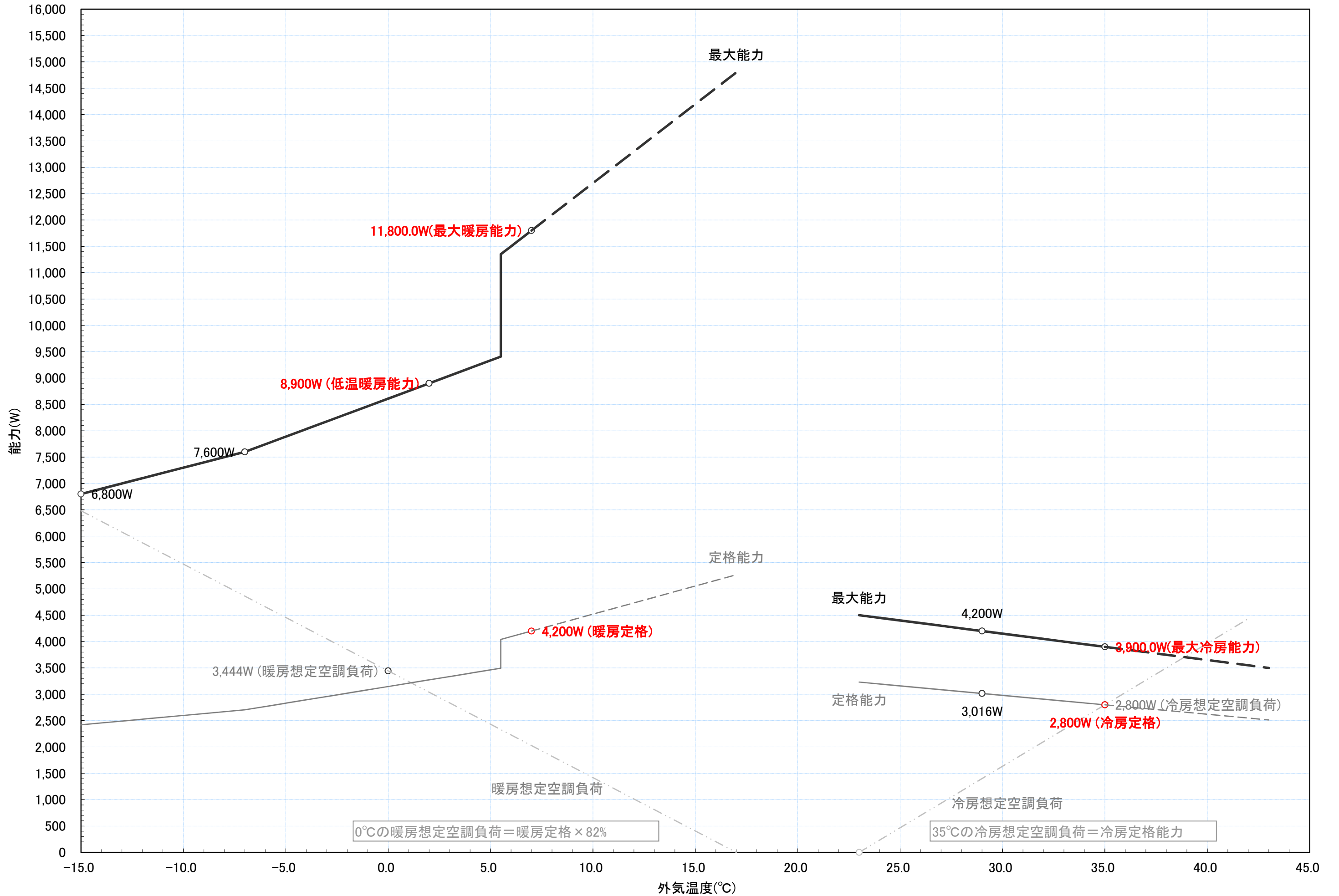
RAS-XK28H2 冷暖房能力特性図 [室温 冷房:27°C一定, 暖房:20°C一定]
