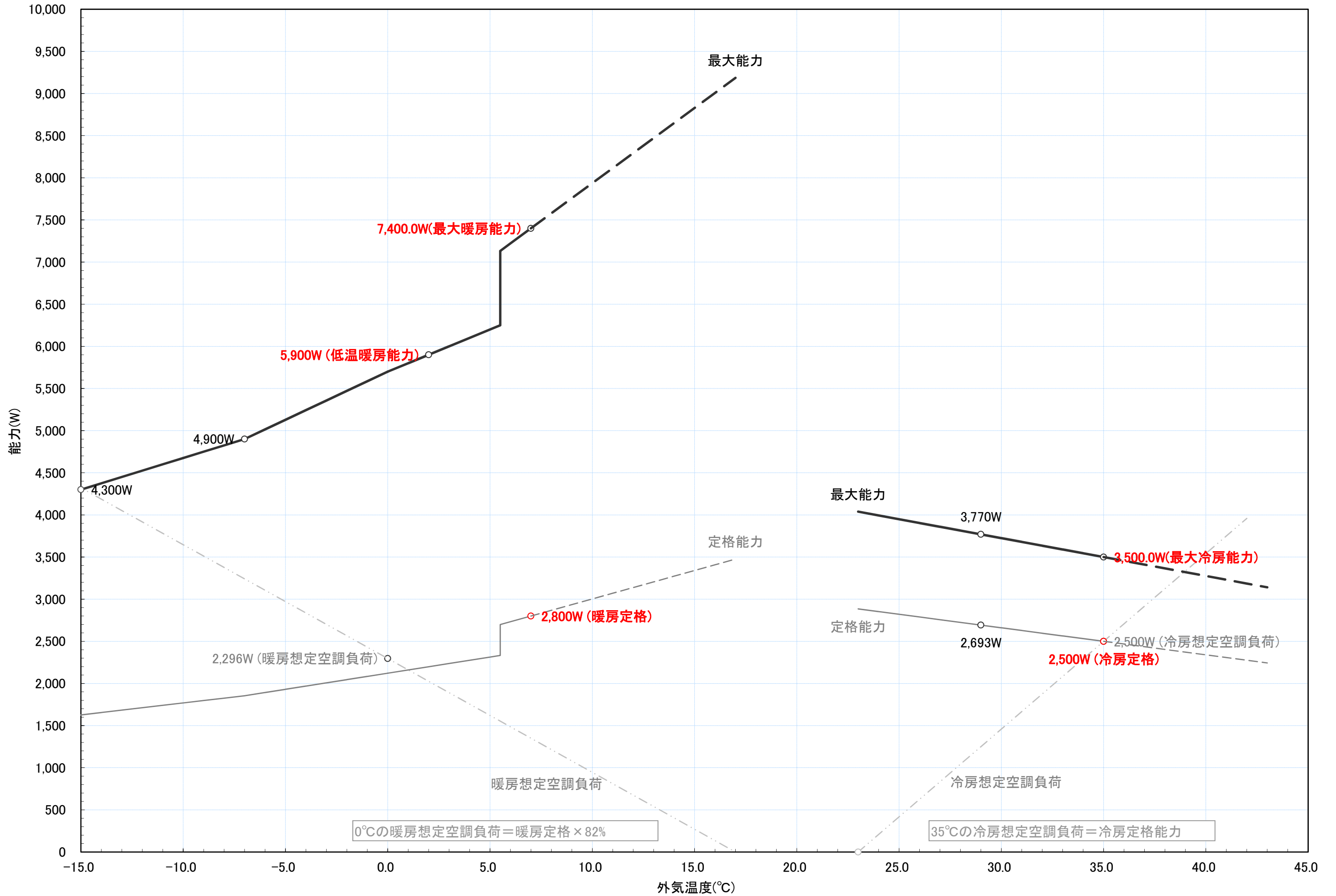
RAS-XK25H 冷暖房能力特性図 [室温 冷房:27°C一定, 暖房:20°C一定]
