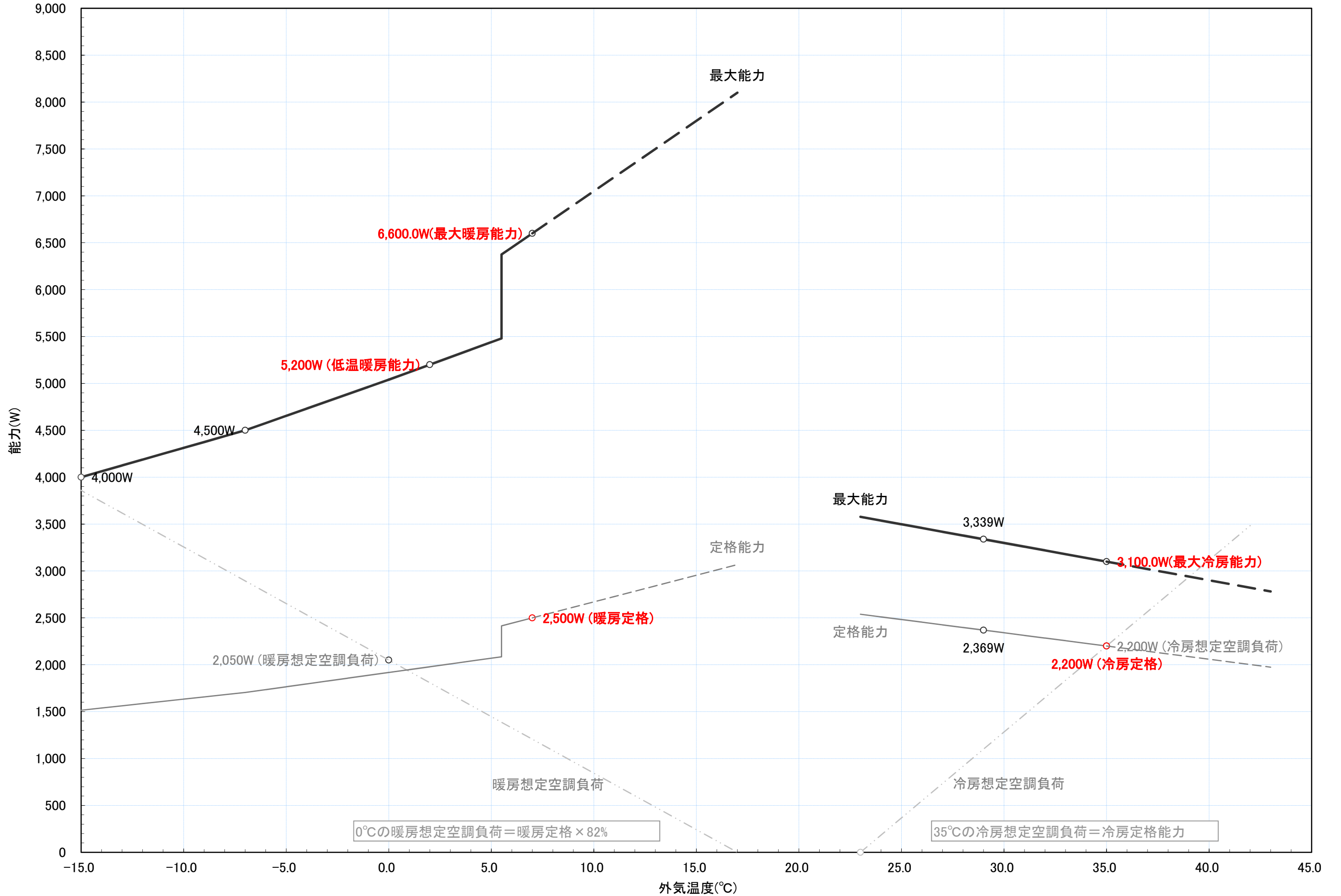
RAS-HK22H 冷暖房能力特性図 [室温 冷房:27°C一定, 暖房:20°C一定]
