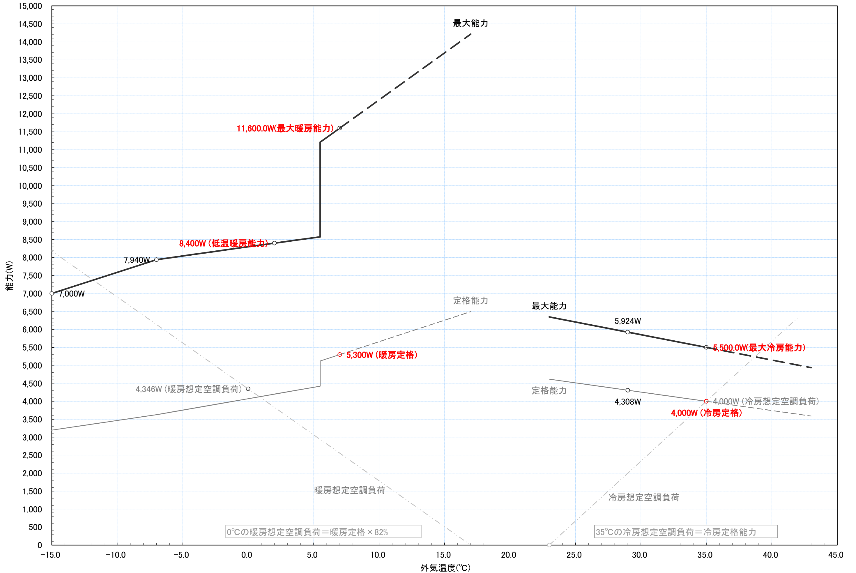
RAS-EK40H2 冷暖房能力特性図 [室温 冷房:27°C一定, 暖房:20°C一定]
