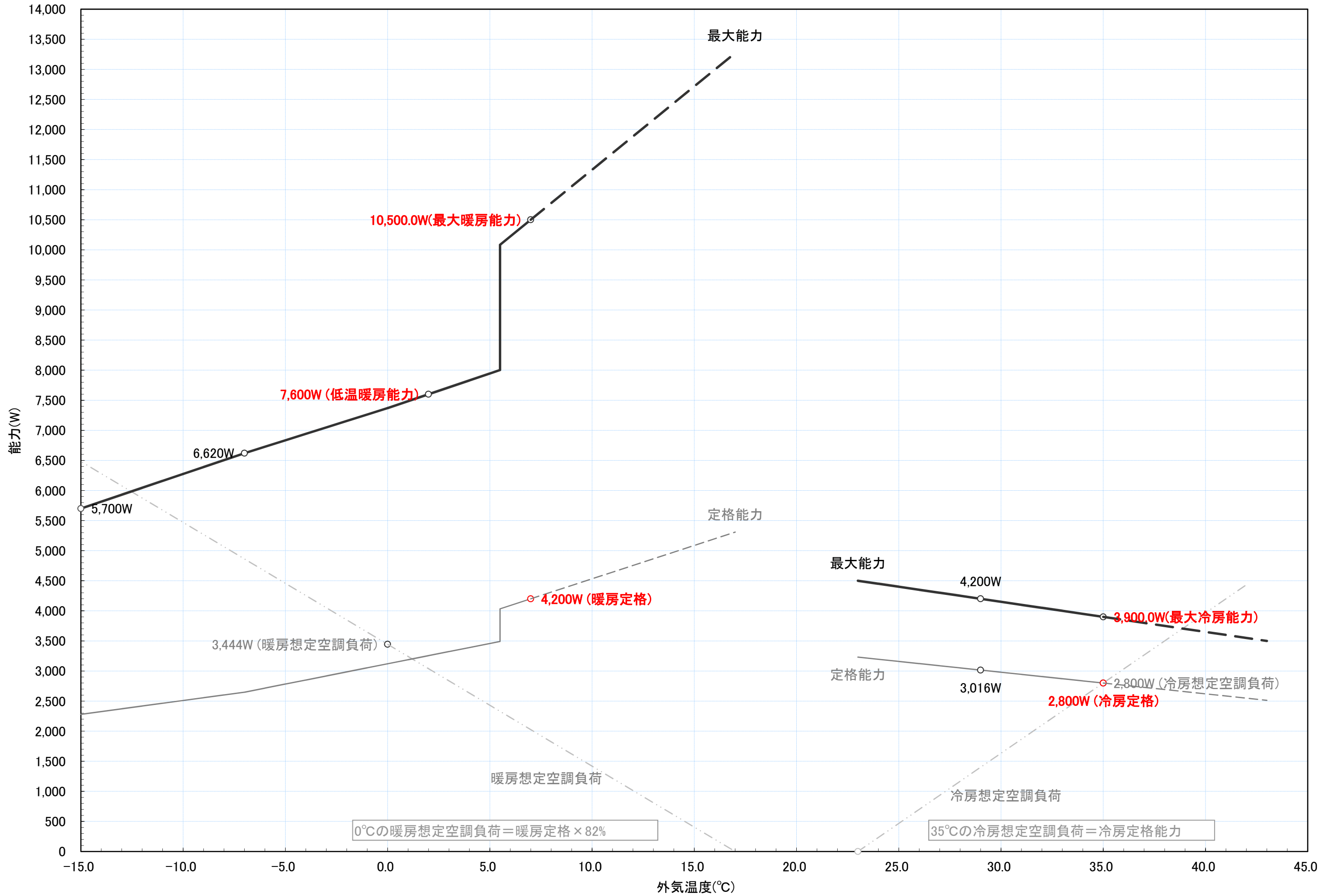
RAS-EK28H2 冷暖房能力特性図 [室温:冷房:27°C一定, 暖房:20°C一定]
