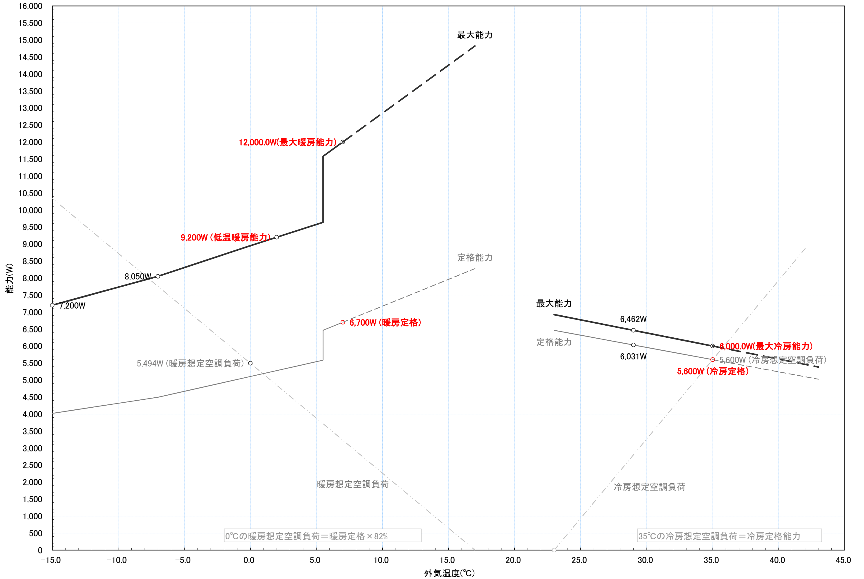
RAS-XK56G2 冷暖房能力特性図 [室温 冷房:27°C一定, 暖房:20°C一定]
