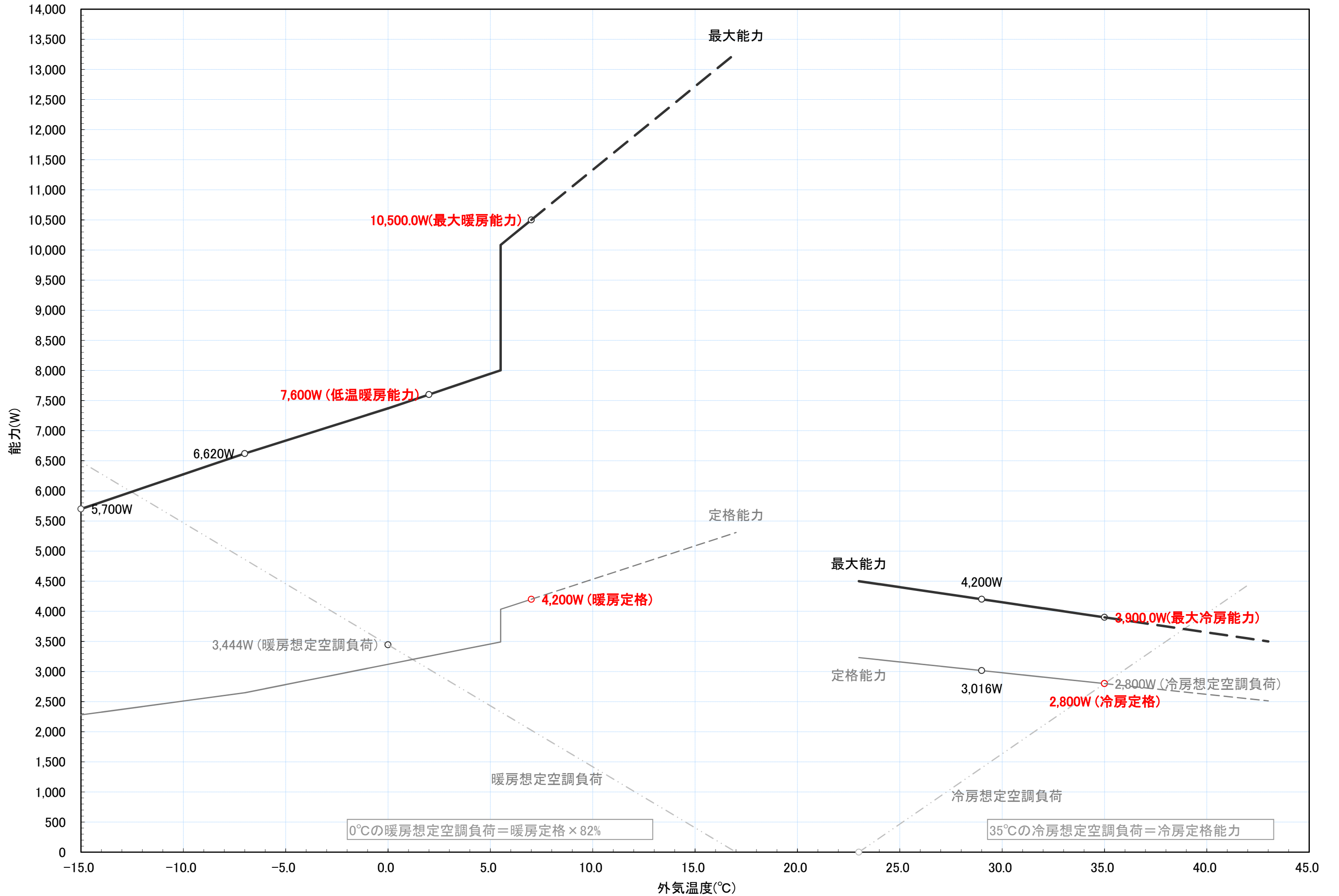
RAS-EK28G2 冷暖房能力特性図 [室温 冷房:27°C一定, 暖房:20°C一定]
