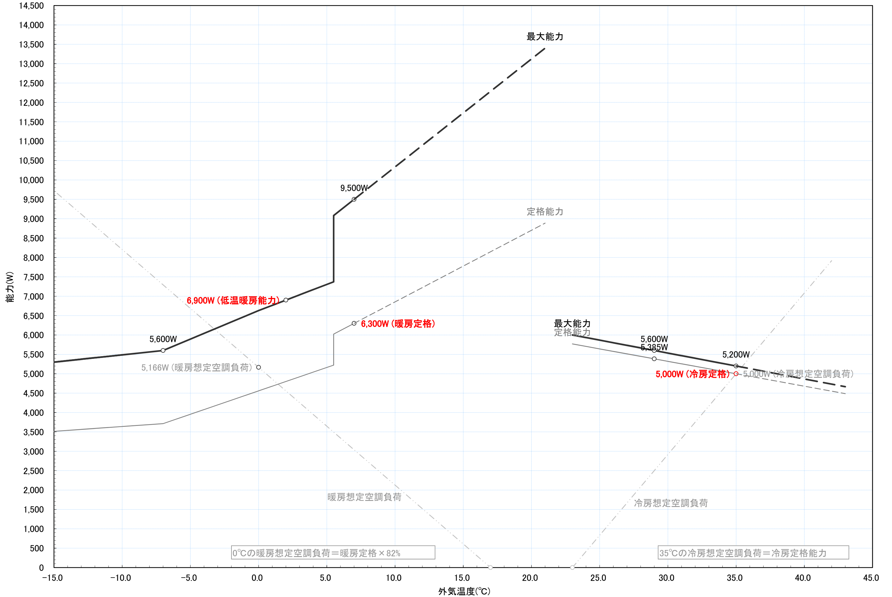
RAF-D50F2 冷暖房能力特性図 [室温 冷房:27°C一定, 暖房:20°C一定]
