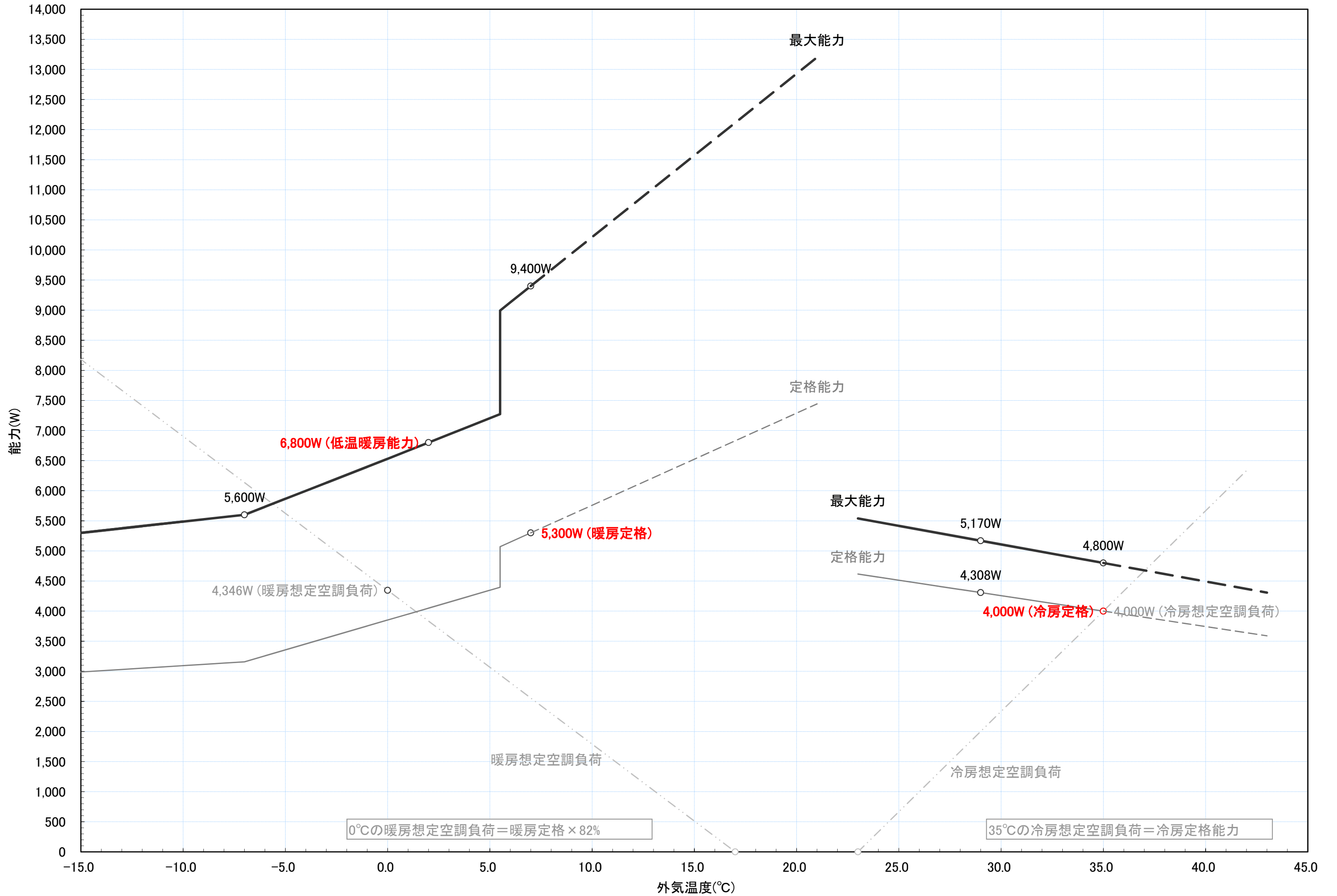
RAF-D40F2 冷暖房能力特性図 [室温:冷房:27°C一定, 暖房:20°C一定]
