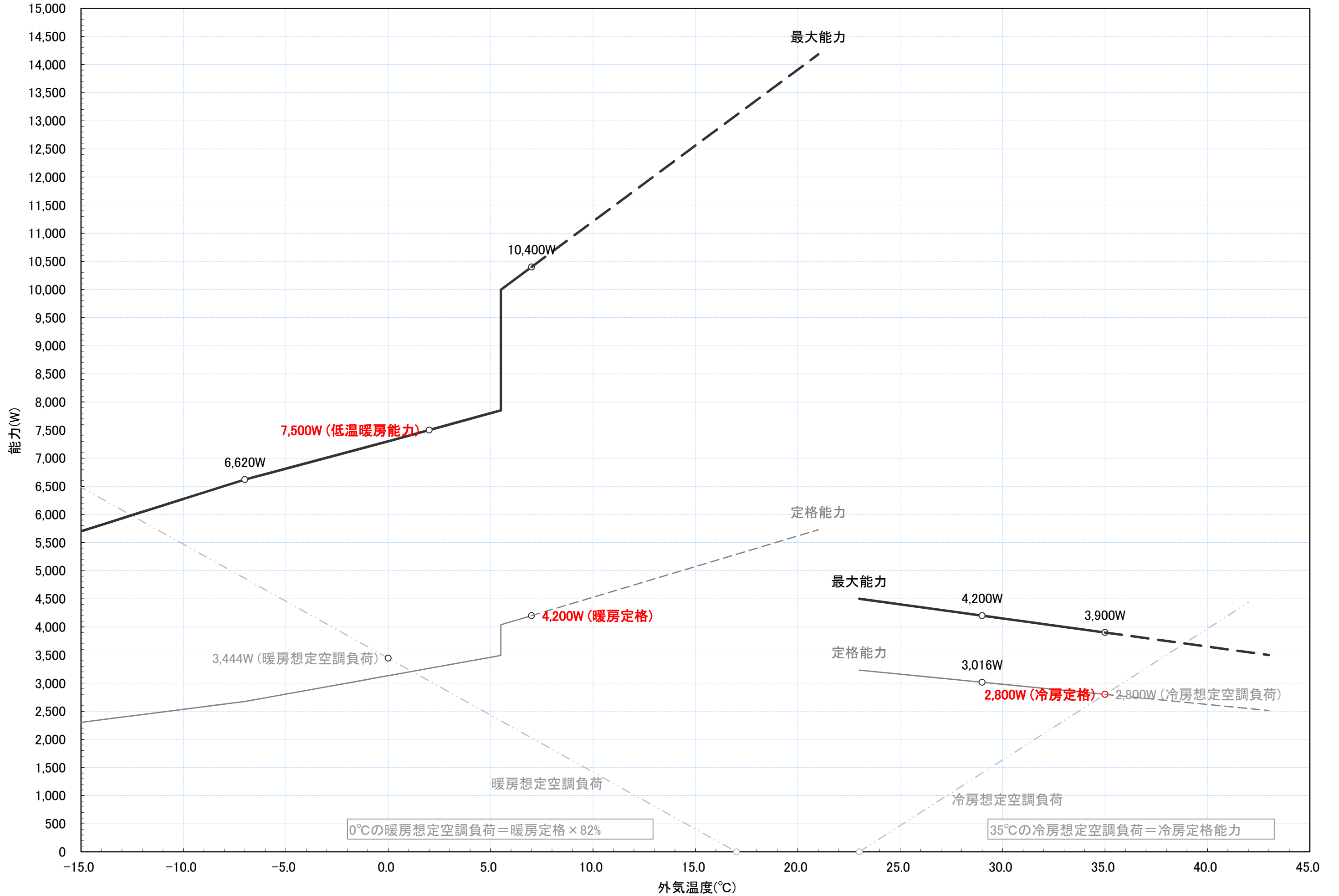
RAS-EK28F2 冷暖房能力特性図 [室温 冷房:27°C一定, 暖房:20°C一定]
