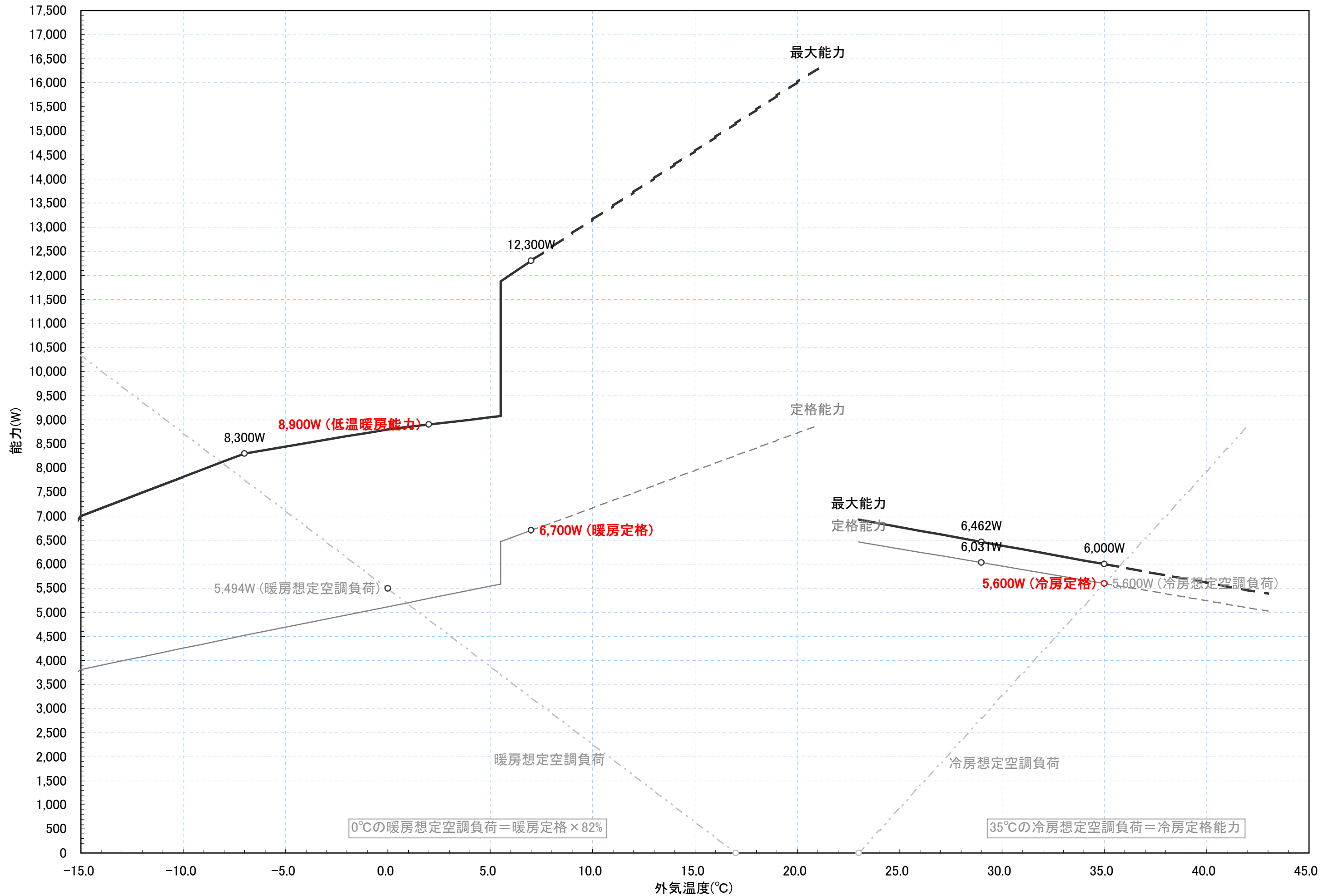
RAS-ZD56E2 冷暖房能力特性図 [室温 冷房:27°C一定, 暖房:20°C一定]
