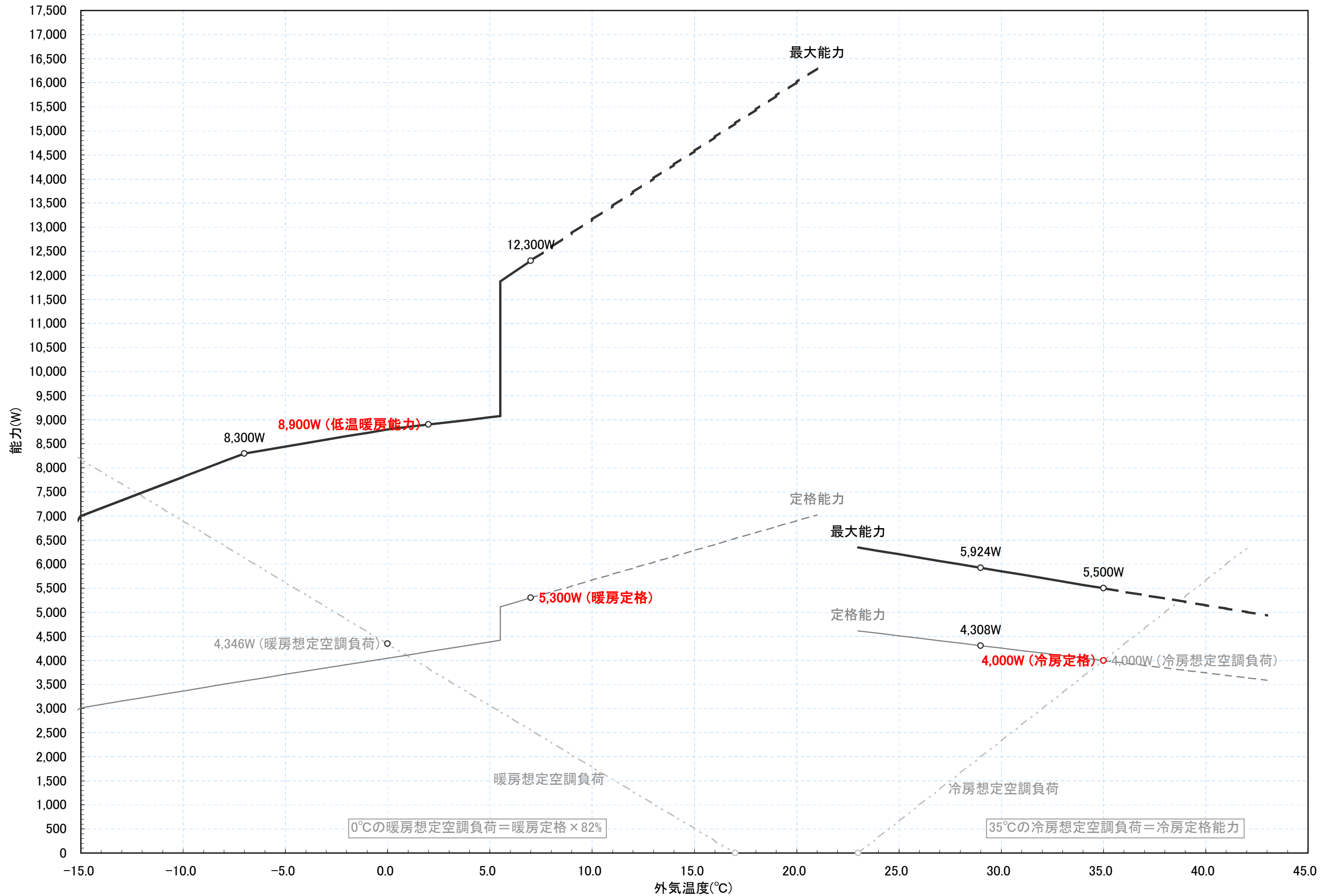
RAS-ZD40E2 冷暖房能力特性図 [室温 冷房:27°C一定, 暖房:20°C一定]
