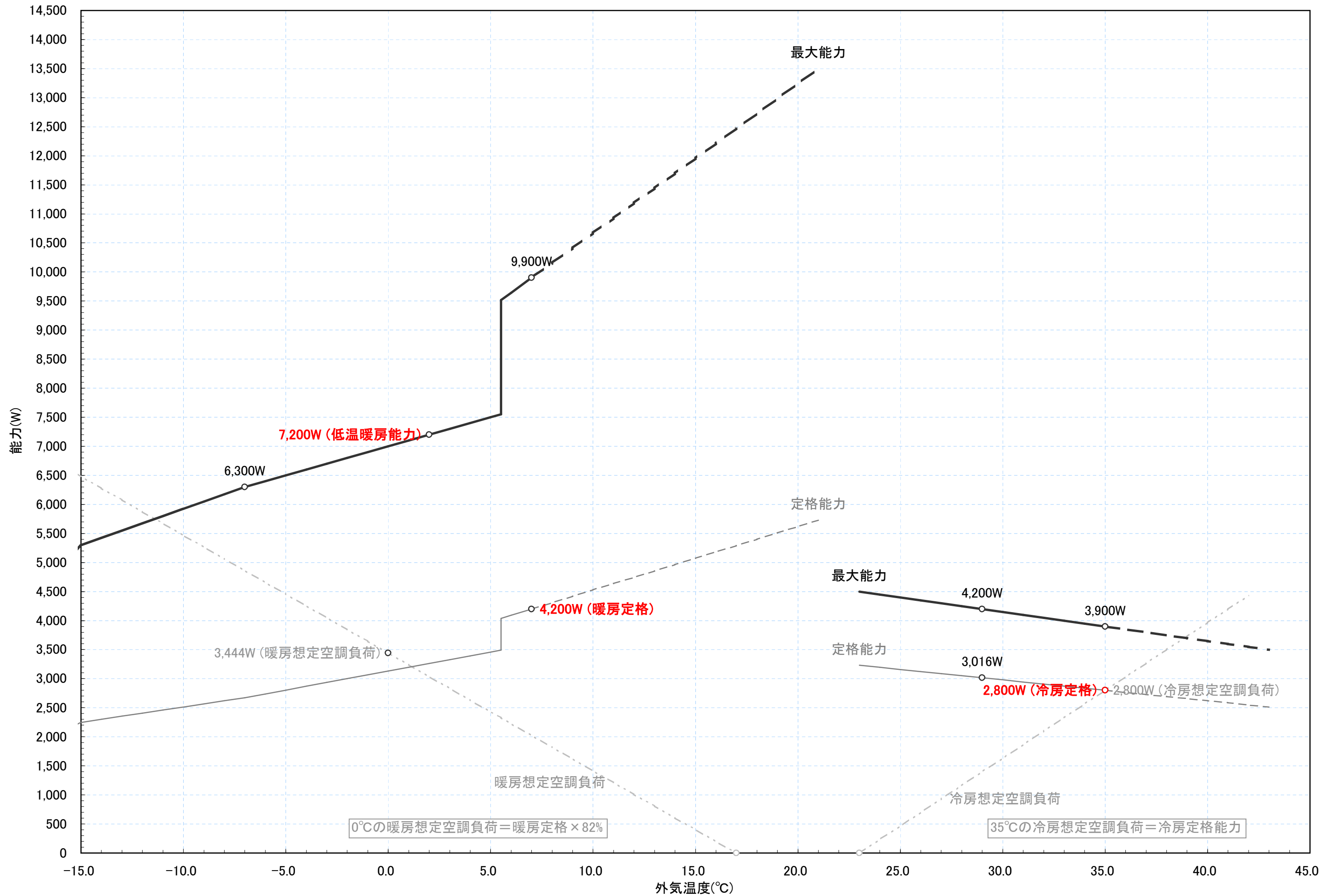
RAS-ZD28E2 冷暖房能力特性図 [室温 冷房:27°C一定, 暖房:20°C一定]
