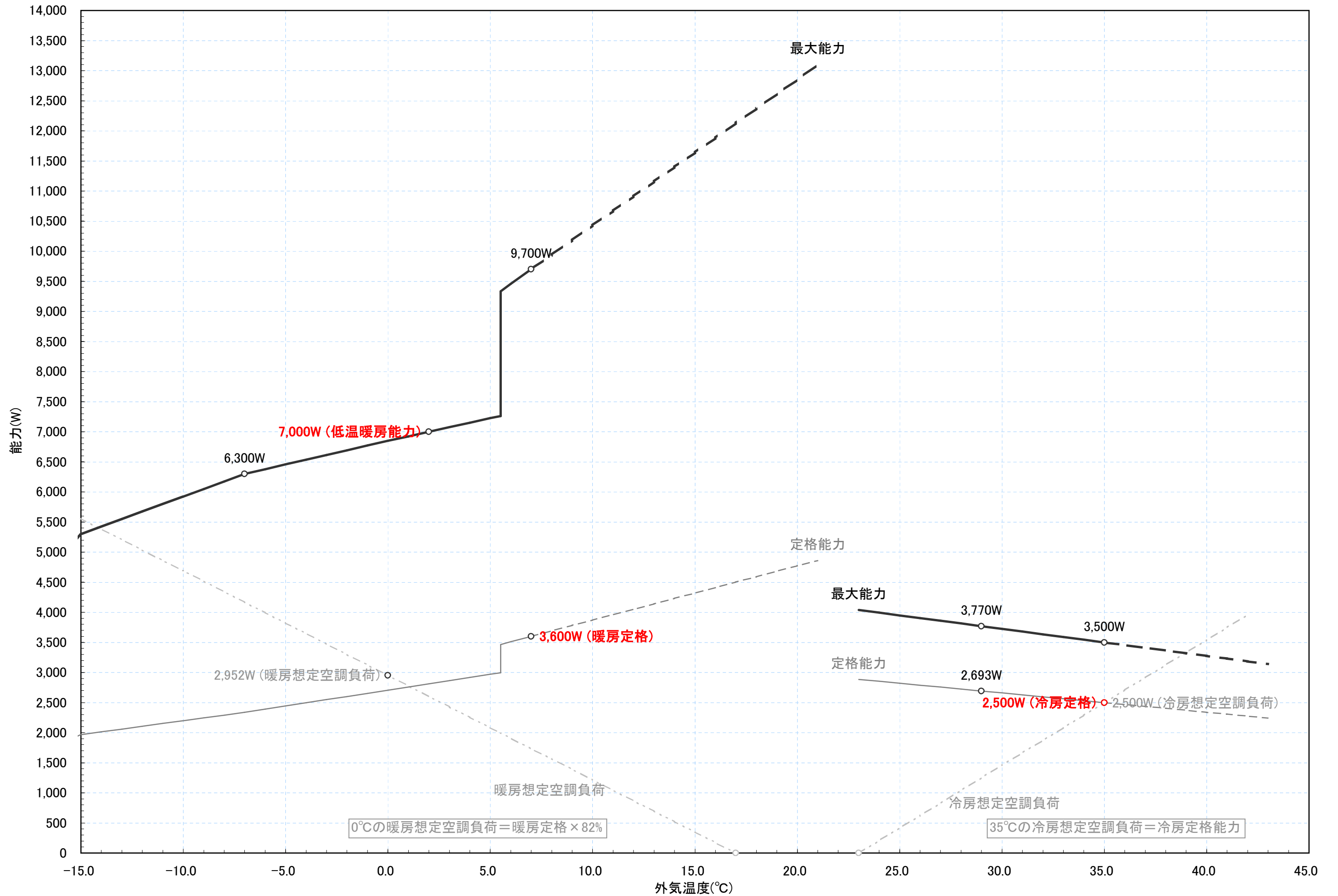
RAS-ZD25E2 冷暖房能力特性図 [室温 冷房:27°C一定, 暖房:20°C一定]
