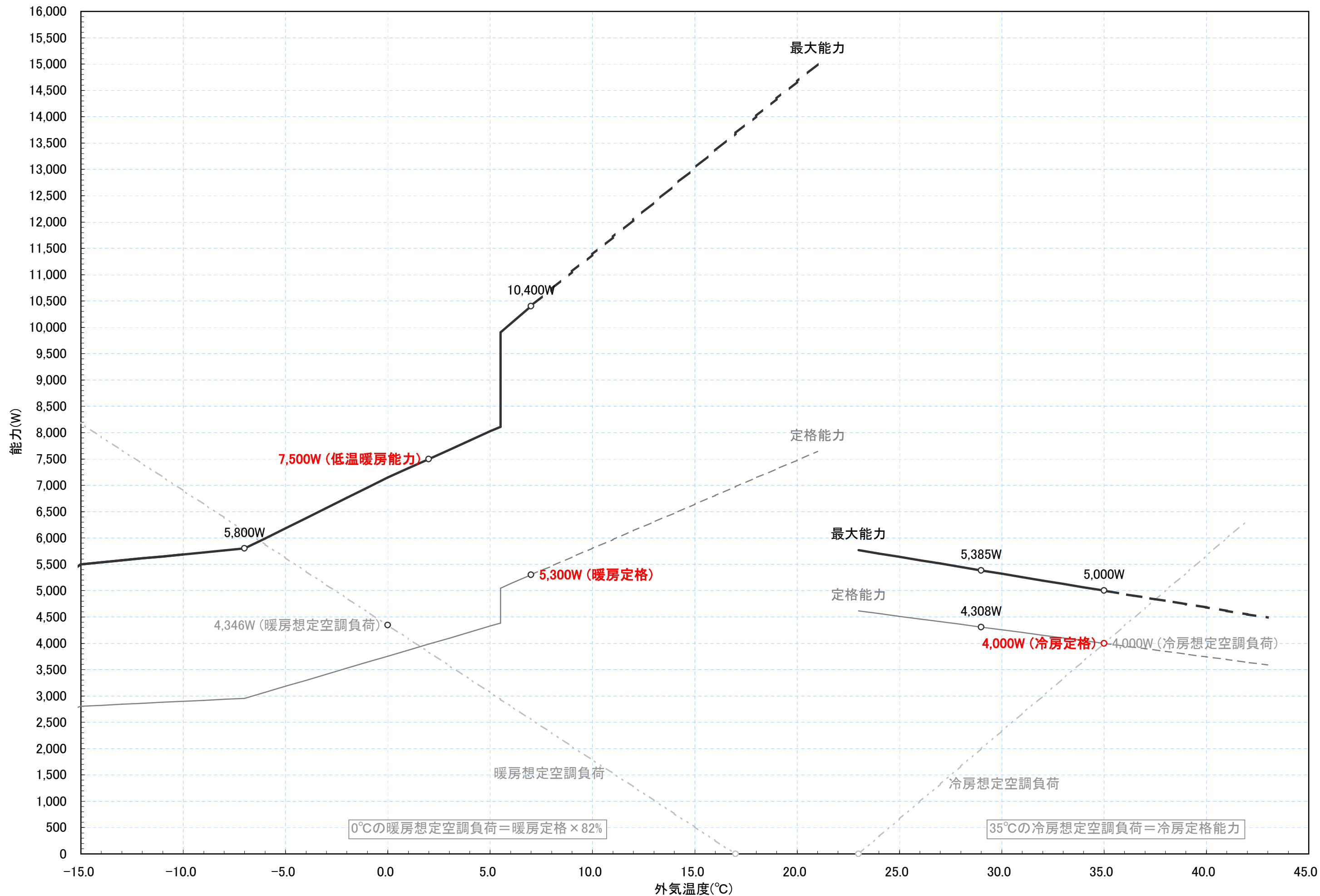
RAS-SD40D2 冷暖房能力特性図 [室温 冷房:27°C一定, 暖房:20°C一定]
