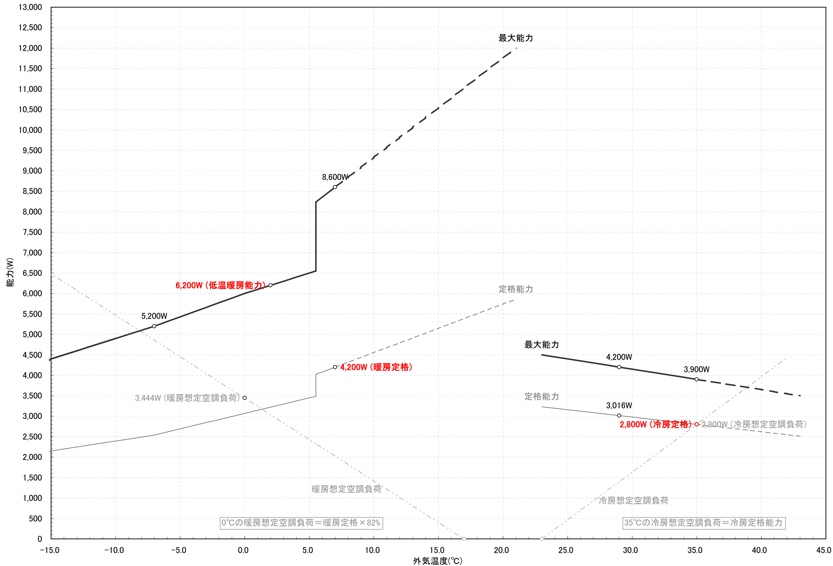
RAS-SD28D2 冷暖房能力特性図 [室温 冷房:27°C一定, 暖房:20°C一定]
