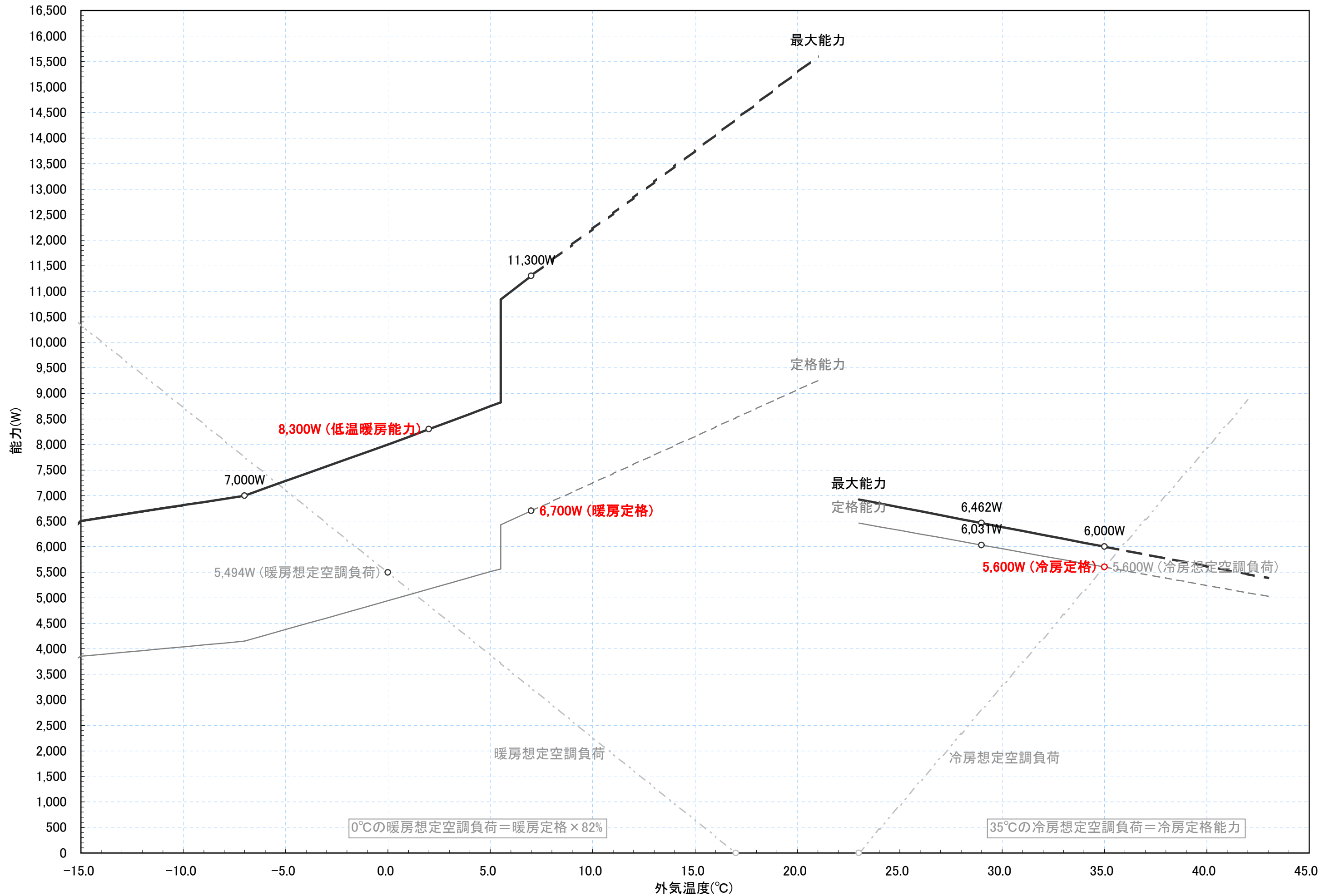
RAS-SK56C2 冷暖房能力特性図 [室温 冷房:27°C一定, 暖房:20°C一定]
