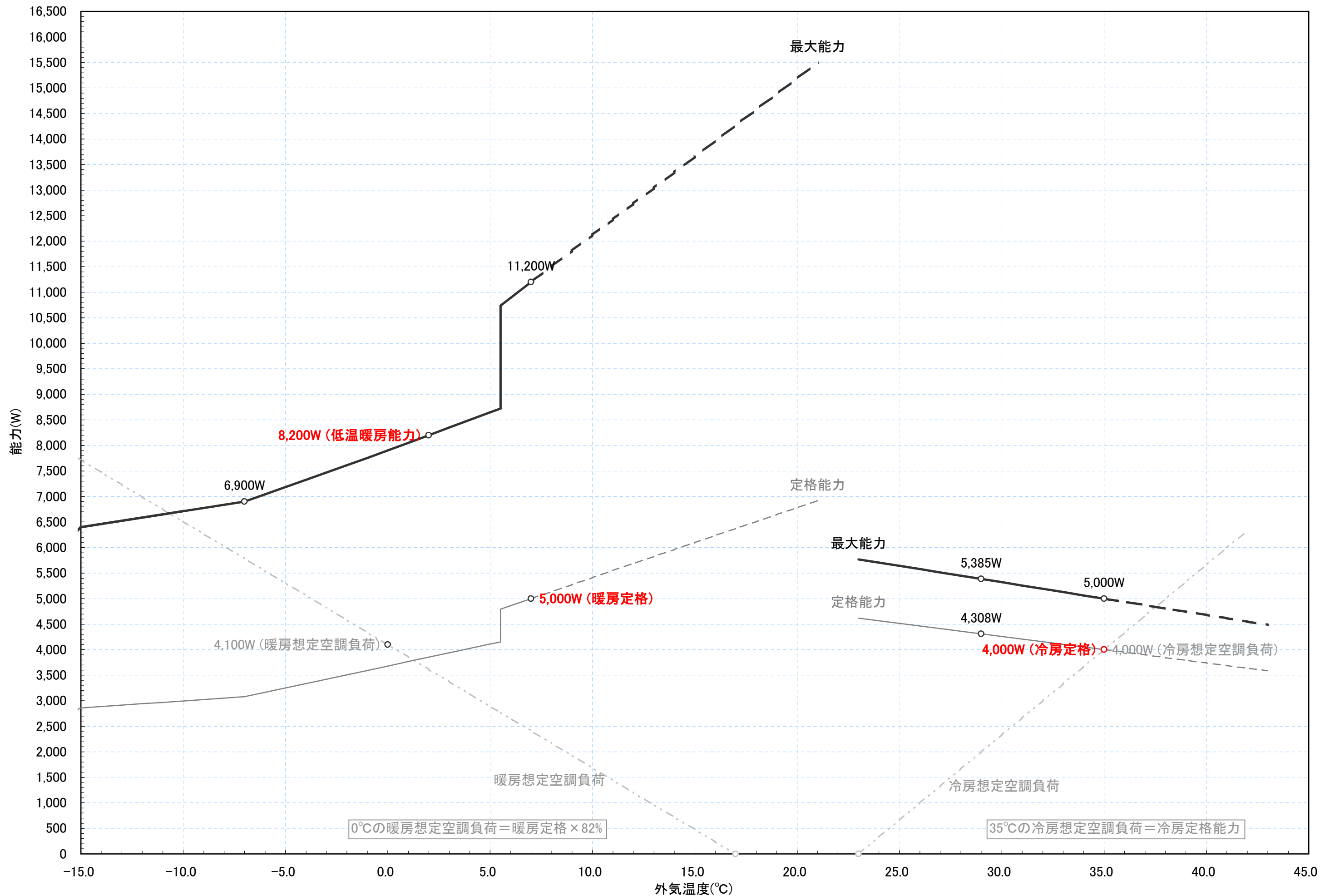
RAS-SK40C2 冷暖房能力特性図 [室温 冷房:27°C一定, 暖房:20°C一定]
