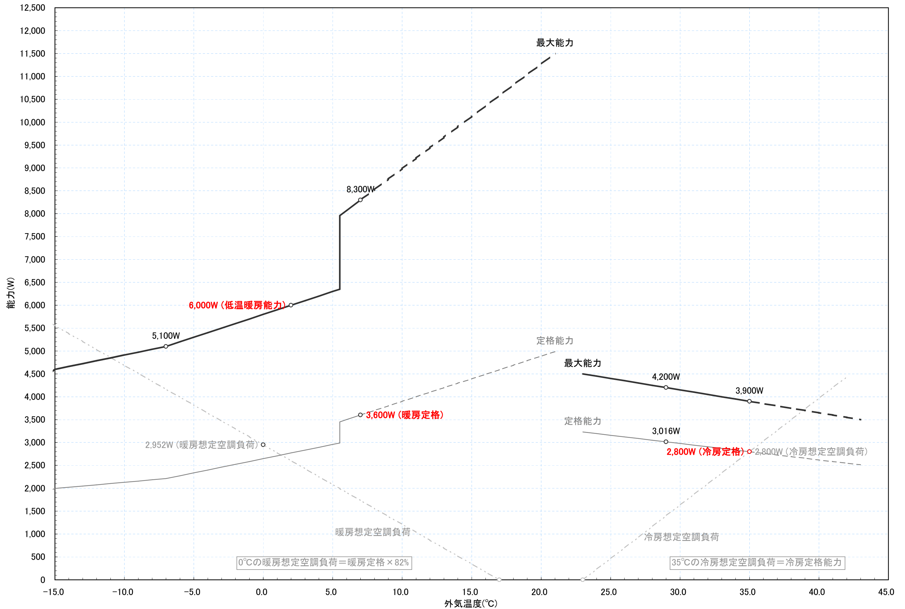
RAS-SK28C2 冷暖房能力特性図 [室温 冷房:27°C一定, 暖房:20°C一定]
