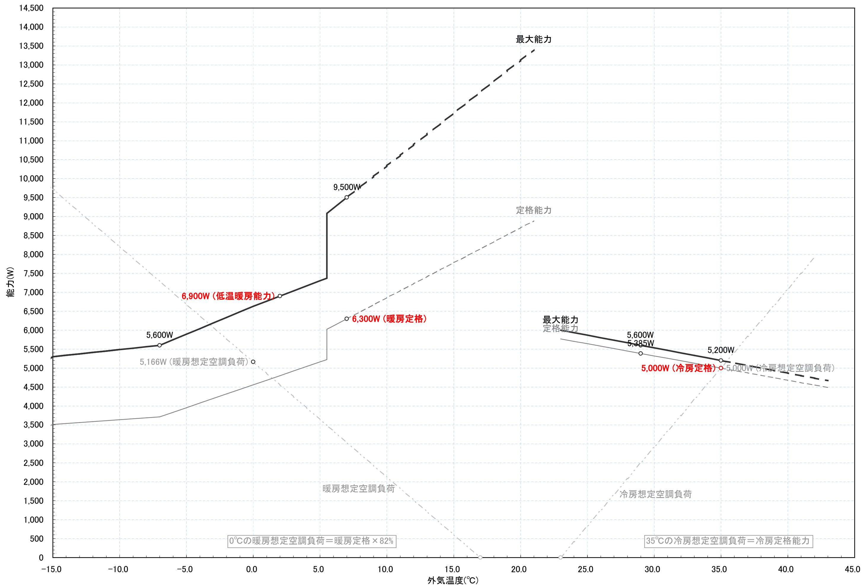
RAF-D50C2 冷暖房能力特性図 [室温 冷房:27°C一定, 暖房:20°C一定]
