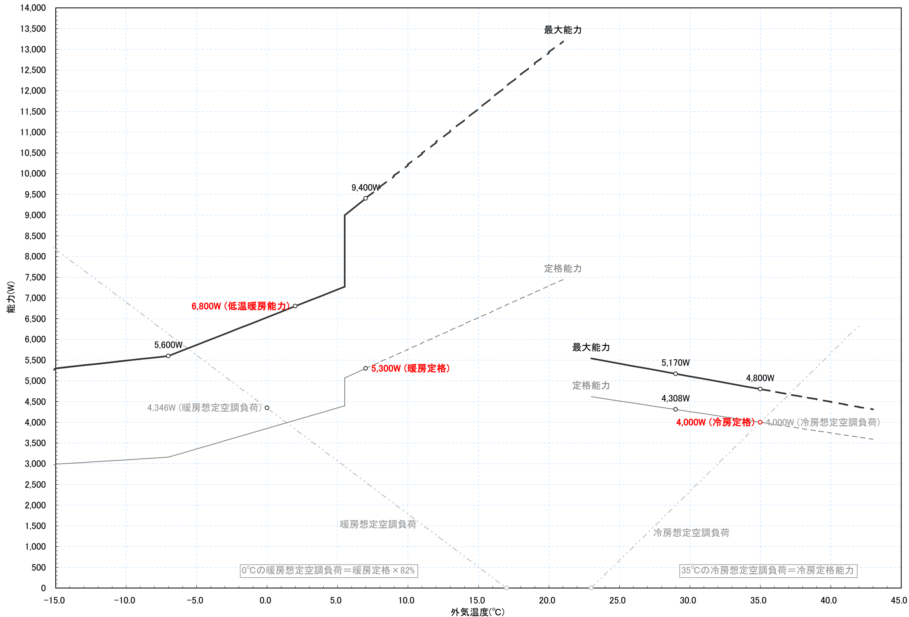
RAF-D40C2 冷暖房能力特性図 [室温 冷房:27°C一定, 暖房:20°C一定]
